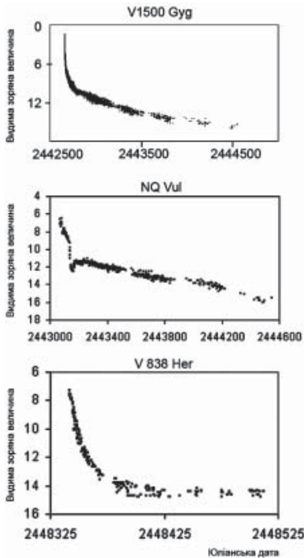
Рис. 17.2. Приклад кривих блиску трьох нових зір V1500 Лебедя, NQ Лисички та V838 Геркулеса, які спалахнули у 1975, 1976 і 1991 роках відповідно
