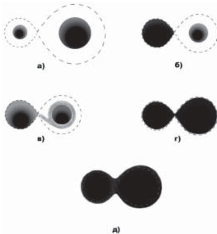
Рис. 15.9. Розділена (а), напіврозділена (б), напіврозділена з газовим потоком між компонентами (в), контактна (г) і надконтактна (д) тісні подвійні системи. Штрихова лінія вказує межі порожнини Роша
