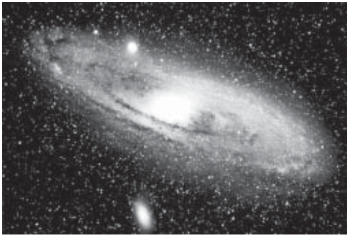
Рис. 20.12. Галактика Туманність Андромеди
