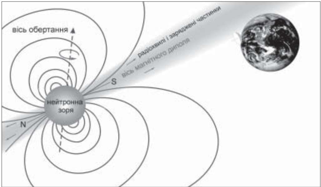
Рис. 17.8. Модель пульсара типу «маяка»
