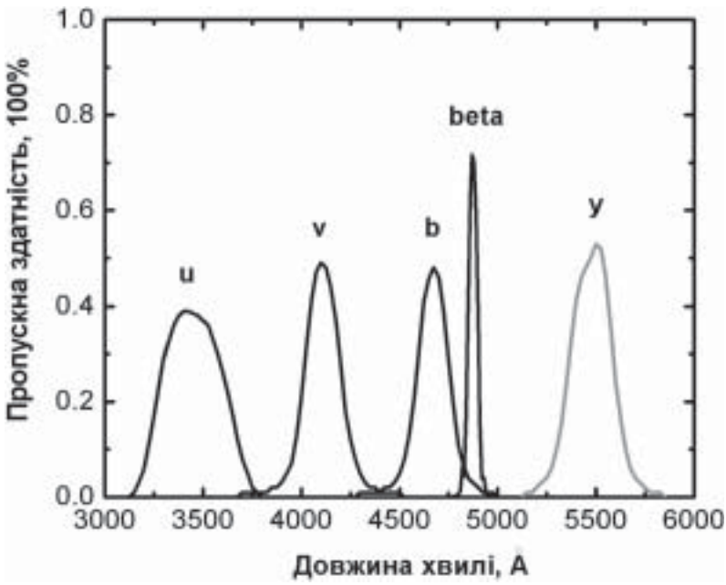
Рис. 8.3. Криві пропускання фільтрів системи UBV (a) і uvbyβ (б)
