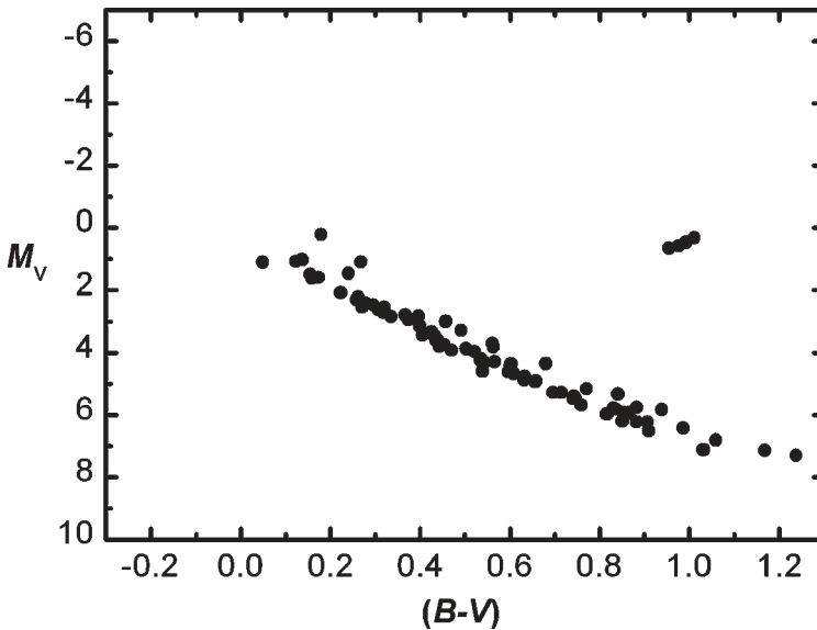
Рис. 19.6. Діаграма колір — зоряна величина для Гіад
