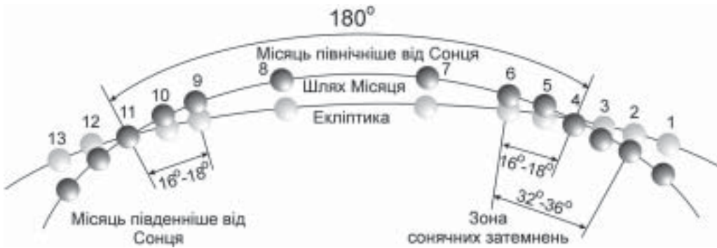
Рис. 5.8. Положення Місяця і Сонця у різні новомісяччя
