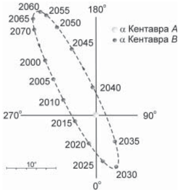
Рис. 15.2. Видима орбіта візуально-подвійної зорі \alpha Кентавра з періодом 79,92 років. Положення компонента B відносно компонента A дається на декілька наступних десятиліть років
