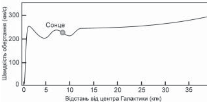
Рис. 19.8. Розподіл швидкостей обертання зір і газу у диску Галактики
