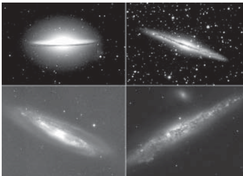
Рис. 20.5. Приклади спіральних галактик, видних із «ребра» (зліва направо): NGC 4594 , NGC 891 , NGC 4192 і NGC 4631
