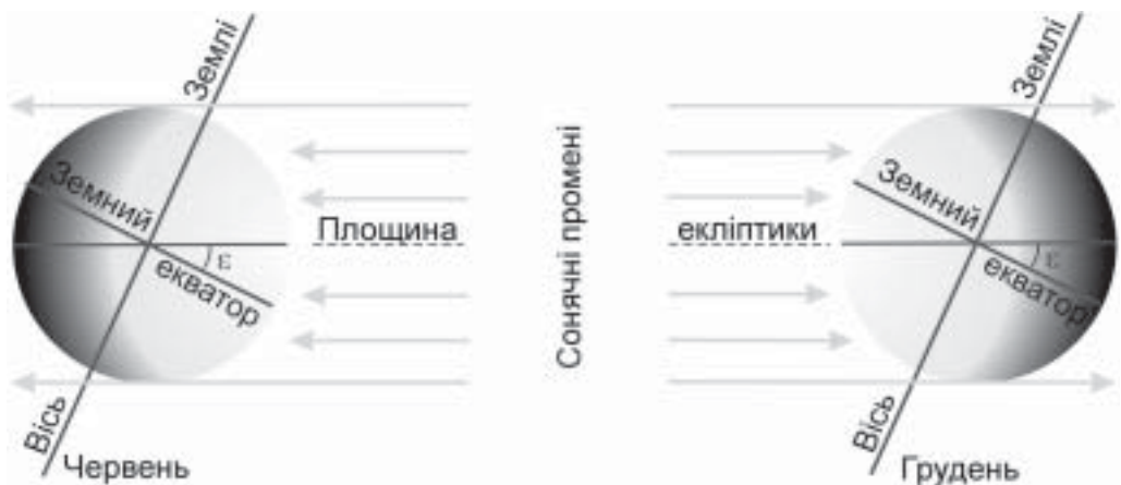
Рис. 2.3. Орбітальний рух Землі навколо Сонця і зміна пір року
