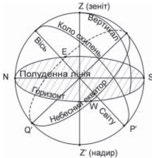
Рис. 1.3. Точки і лінії небесної сфери
