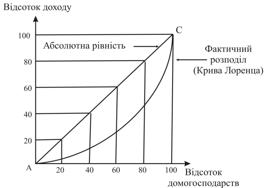
Рис. 2.1. Крива Лоренца
