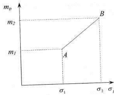
Рис.1. Множина портфельів двох абсолютно додатньо корельованих видів акцій
