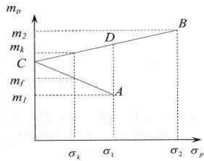
Рис. 2. Множина портфелів з двох абсолютно від'ємно корельованих видів акцій
