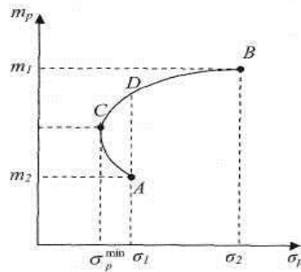
Рис. 3. Множина портфелів двох некорельованих видів акцій
