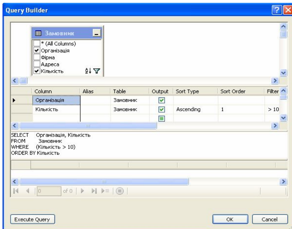
Рисунок 6.18 – Створення SQL -запиту
