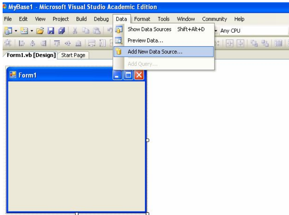
Рисунок 6.5 – Виклик майстра ADO.NET для з'єднання з БД
