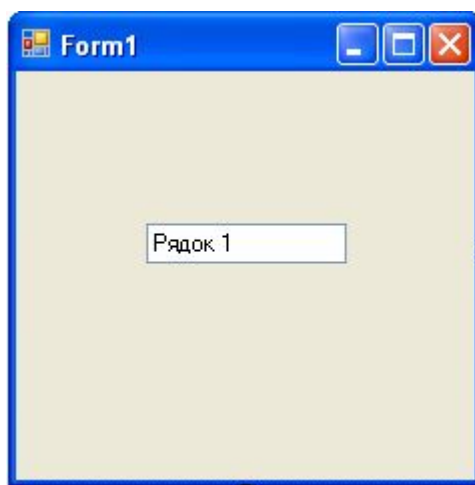
Рисунок 3.2 – ЕК TextBox
