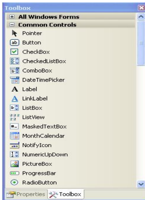
Рисунок 3.1 – Вікно Toolbox
