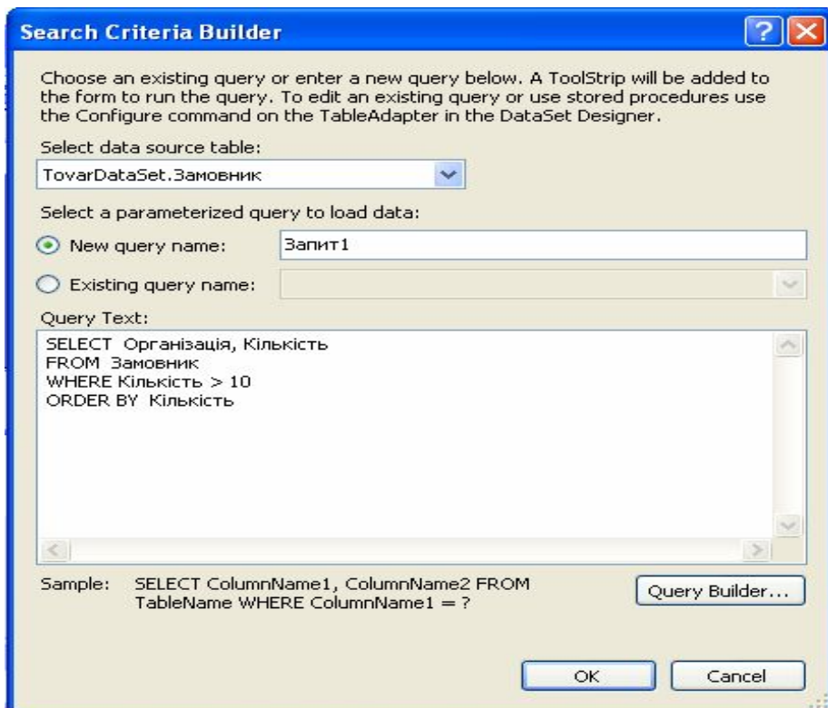
Рисунок 6.17 – Виклик майстра для створення SQL -запитів
