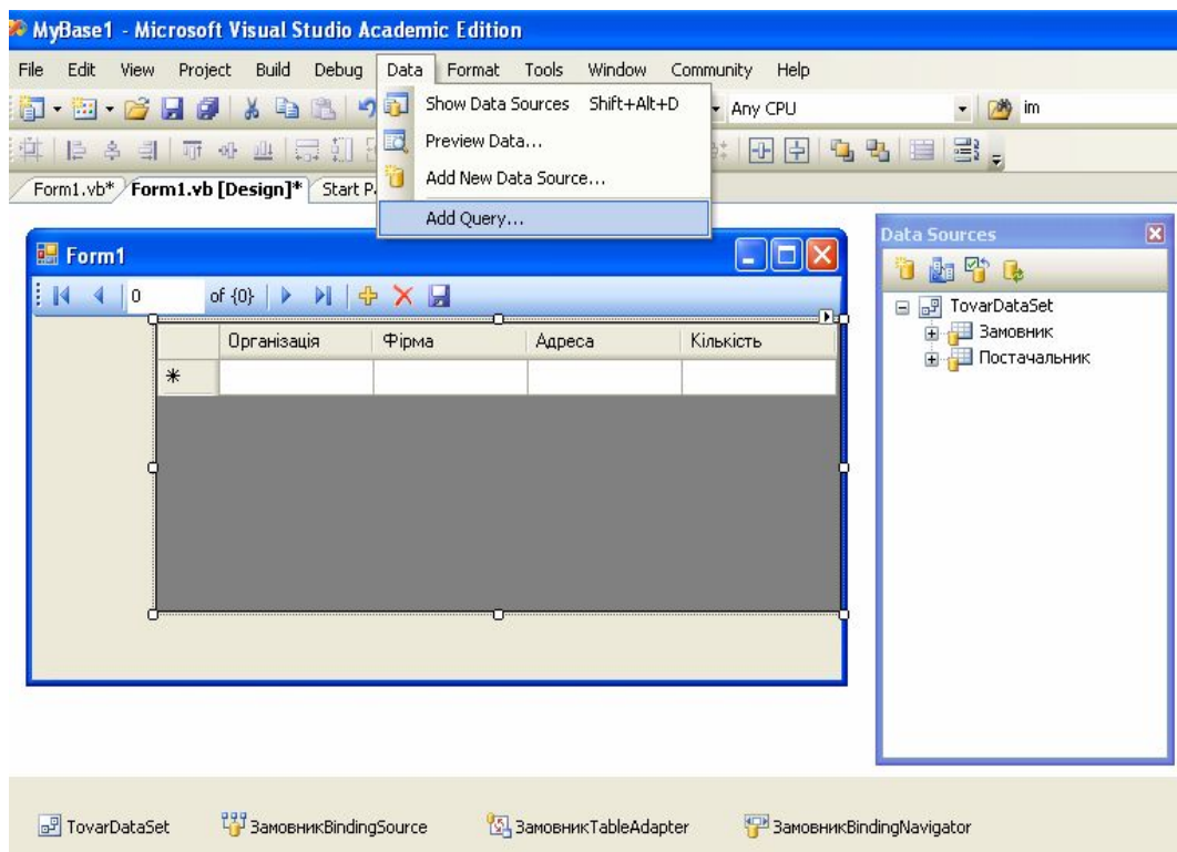
Рисунок 6.16 – Виклик майстра для створення SQL -запитів
