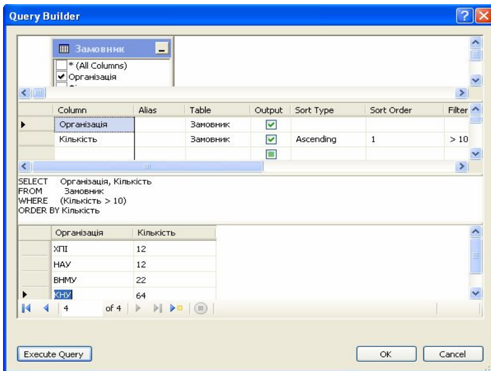
Рисунок 6.19 – Результат виконання SQL -запиту
