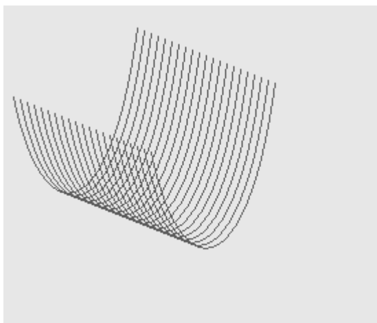
Рисунок 4.2 – Криві Без'є
