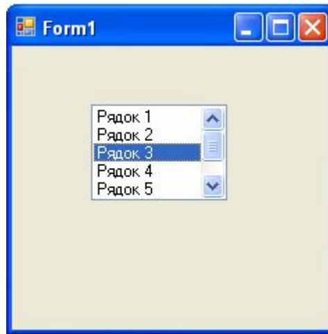
Рисунок 3.6 – ЕК ListBox
