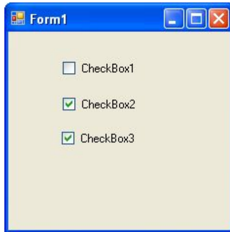
Рисунок 3.4 – ЕК CheckBox
