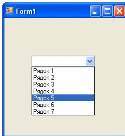
Рисунок 3.7 – ЕК ComboBox
