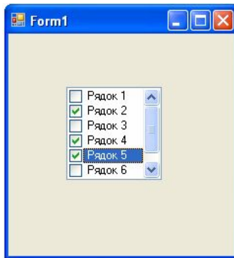
Рисунок 3.8 – CheckedListBox
