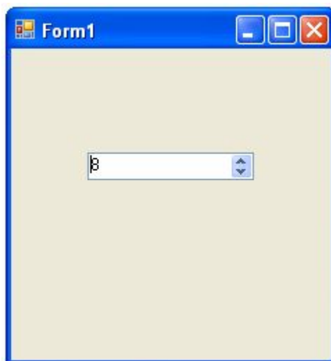
Рисунок 3.9 – NumericUpDown
