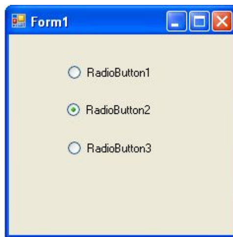
Рисунок 3.5 – ЕК RadioButton
