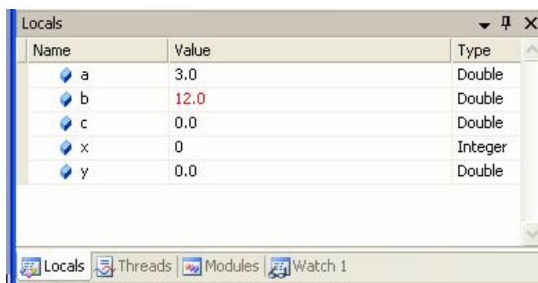
Рисунок 5 – Вікно Locals
