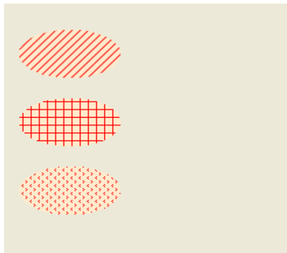
Рисунок 4.4 – Приклади штриховки
