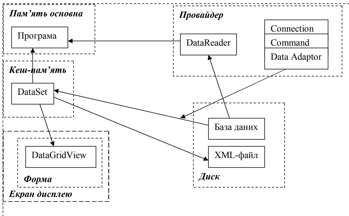
Рисунок 6.1 – Архітектура ADO.NET
