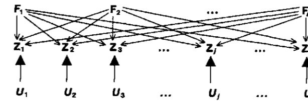
Рис. 7.1. Схема соотношений между наблюдаемыми признаками ( z_1, \dots, z_n ) и латентными факторами: общими ( F_1, \dots, F_m ) и специфическими ( U_1, U_2, \dots, U_n )
