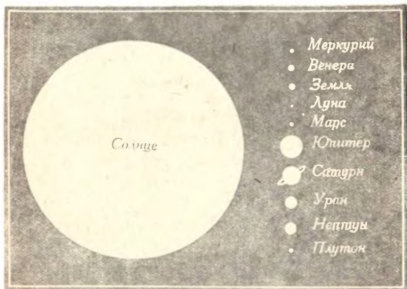
Рис. 7. Сравнительные размеры Солнца и планет.
