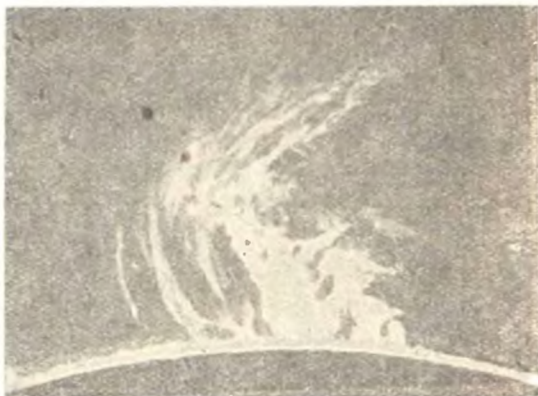
Рис. 2. Протуберанцы Солнца.
