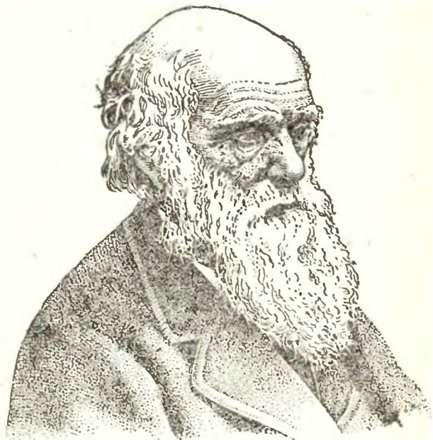
Рис. 30. Чарлз Дарвин (1809)—1882).
