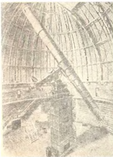
Рис. 1. Телескоп.
