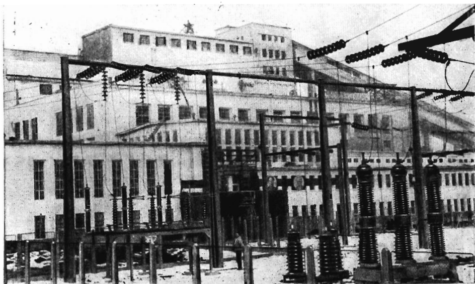
ТЭЦ «Республика» близ города Димитрово
