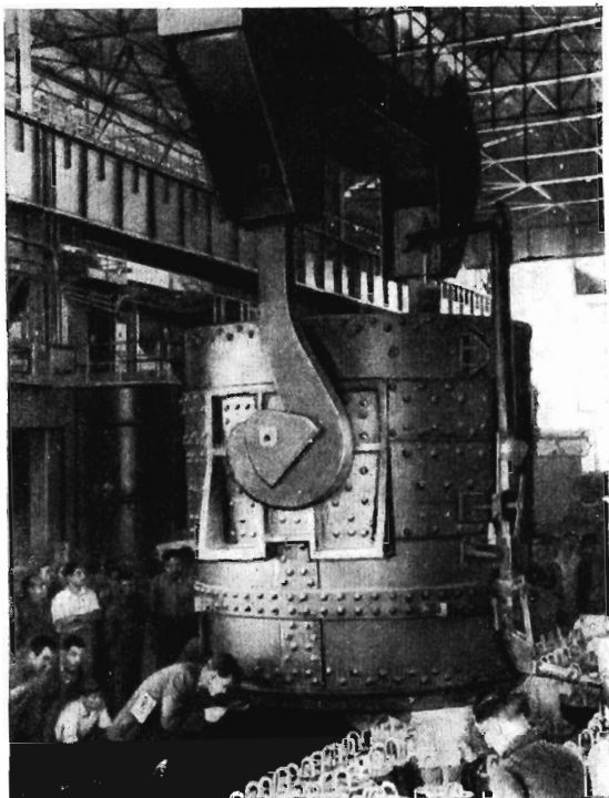
Разлив первой стали на металлургическом заводе имени В. И. Ленина восточнее г. Димитрово
