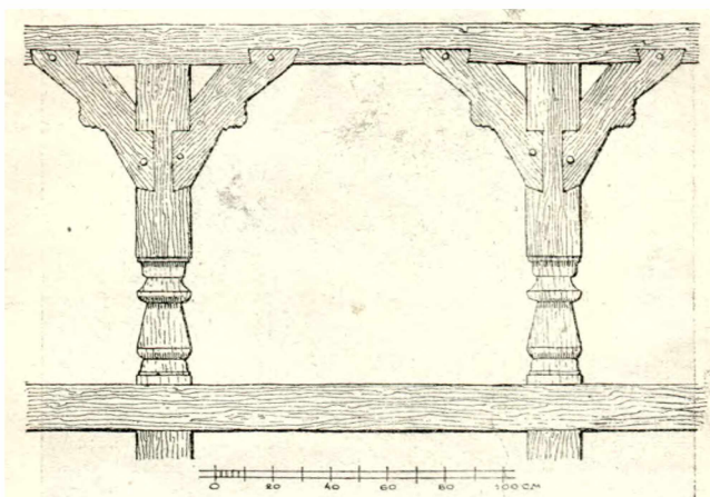
Рис. 27. С. Плоске. Церква 1790-их рок. Сохи опорання.
