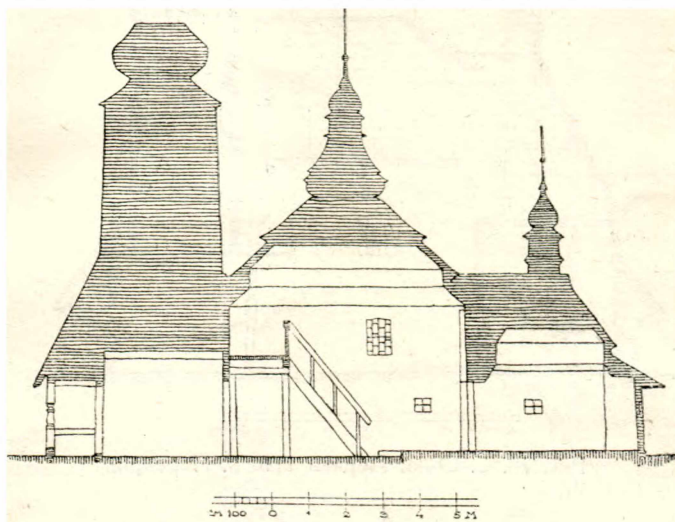
Рис. 26. С. Плоске. Церква 1790-их рок. Перекрій.
