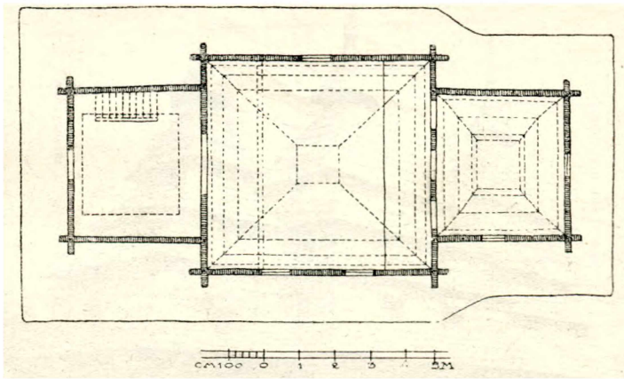
Рис. 9. С. Кострини. Церква 1761 р. Плян.
