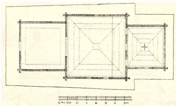
Рис. 14. С. Суха. Церква 1769 р. Плян.
