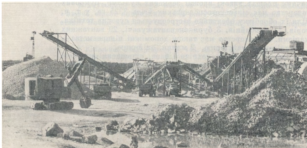
Добування граніту в кар'єрі № 3. Рокитне. 1970 р.
