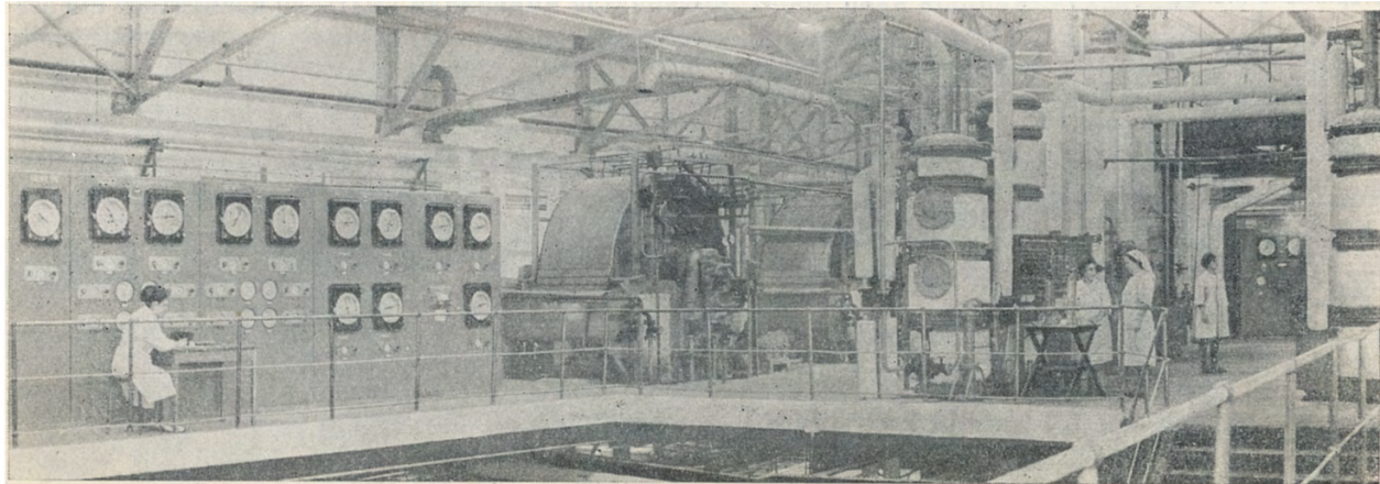
Загальний вигляд сокоочисного цеху Яготинського експериментального цукрового заводу. 1964 р.
