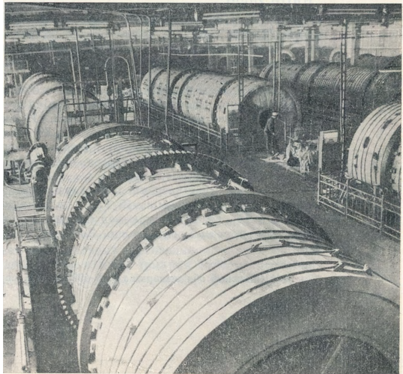
Загальний вигляд напівавтоматичного зольно-дубильного цеху 4-го шкірзаводу, м. Васильків. 1969 р.
