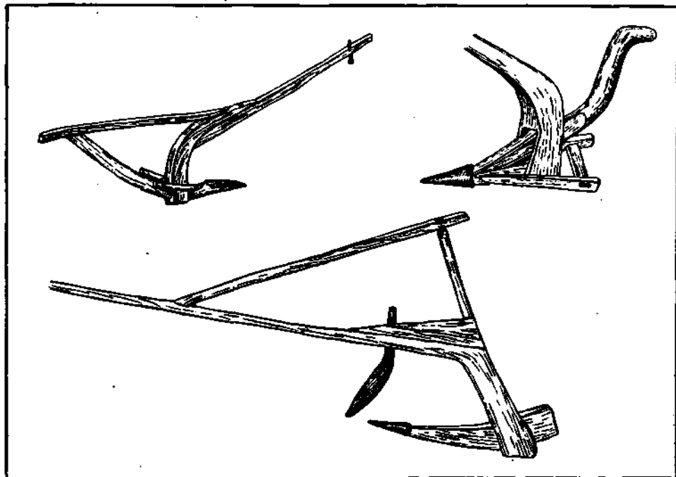
Кривоградильные рала I тысячелетия н. э.: скандинавское (№ 1), балканское (№ 2), шотландское (№ 3)
