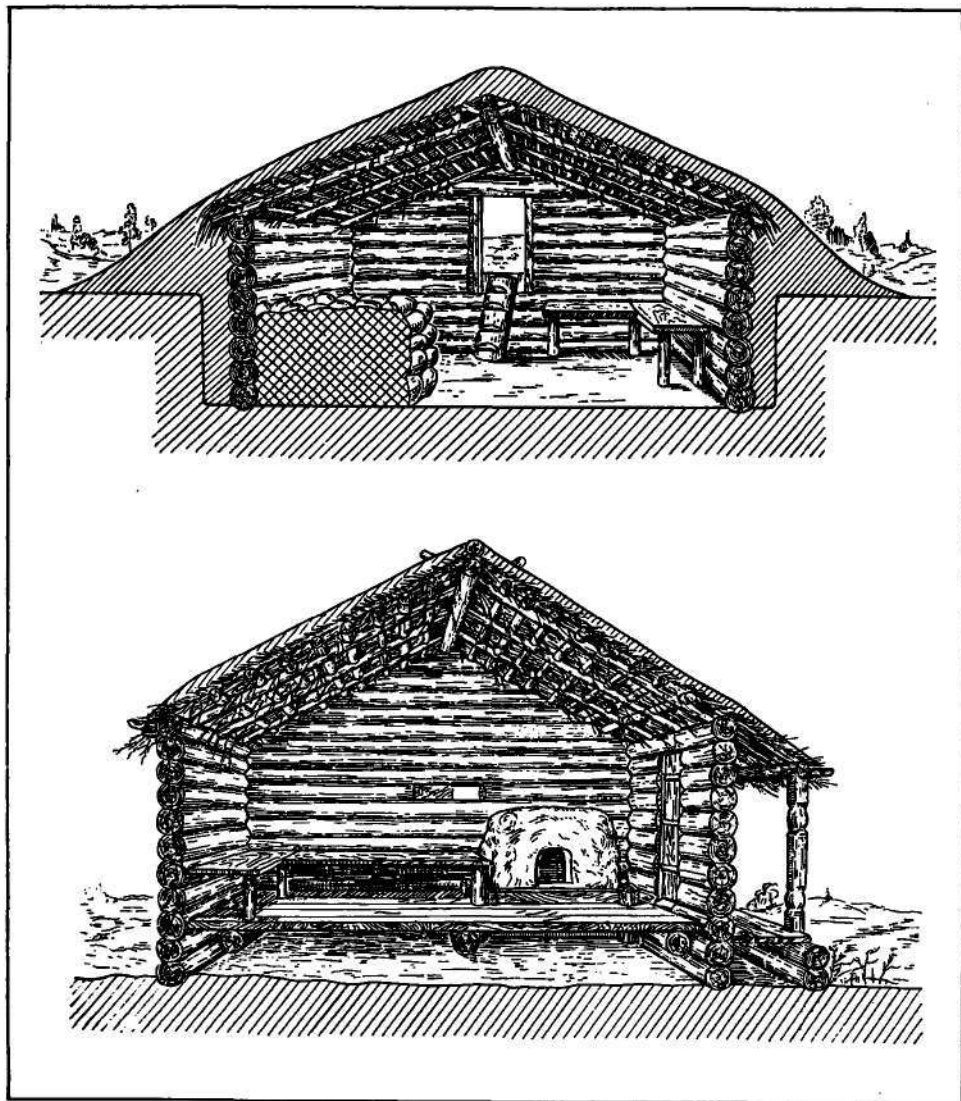
Реконструкция восточнославянской полуземлянки VIII—X вв.
