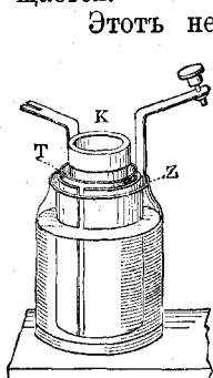
Элементъ Даниеля Т-глиняный сосудъ Z-цинковый цилиндръ, К-мѣдный цилиндръ. См. текстъ на этой стр.
