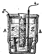
Элементъ Мейдингера. А-стеклянный сосудъ, Z-цинковая пластинка, d-стаканъ, e-листовая мѣль, h-открытая снизу трубка съ мѣднымъ купоросомъ. См. текстъ выше.
