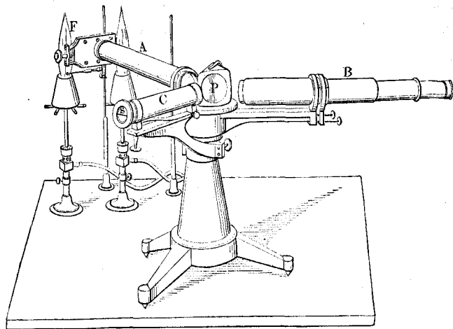
Спектроскопъ Бунзена.
