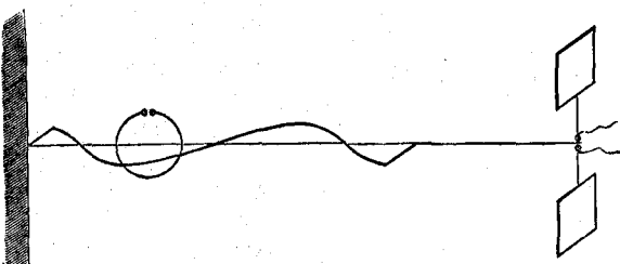
Исслѣдованіе формы электрическихъ волнъ при помощи резонатора Герца. См. текстъ, стр. 360.
