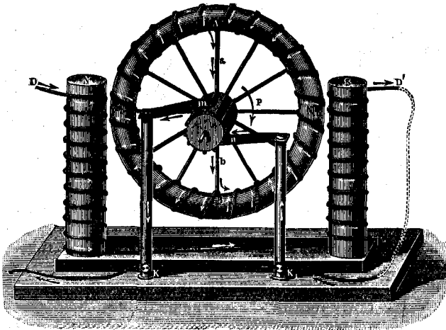
Схема машины постояннаго тока. См. текстъ, стр. 350.
