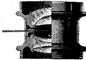
Анастигматъ Цейсса.
