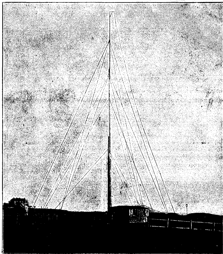
Станція безпроводнаго телеграфа на Гельголандѣ. См. текстъ, стр. 357.
