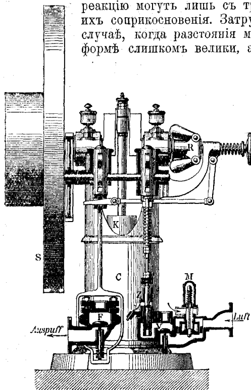
Газовый двигатель. С цилиндръ, К поршень, Z, M, F, V клапаны, R регуляторъ, S маховое колесо. См. текстъ, стр. 173.
