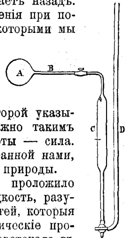
Воздуш- ный тер- мометръ. См. текстъ, стр. 45.
