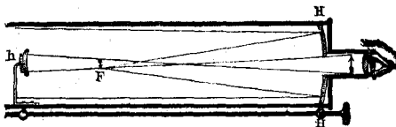
Телескопъ Грегори (рефлекторъ). См. текстъ, стр. 213.
