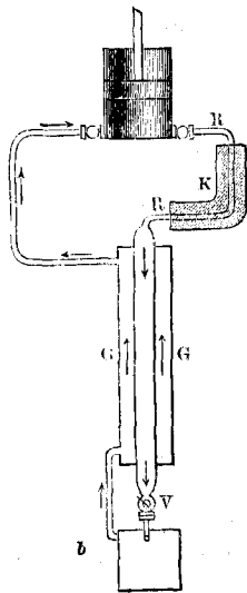
Машина Лиде. в. схематическое изображение.
