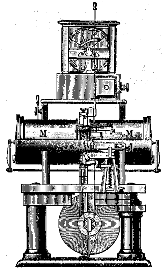
Сифонный самопишущій аппаратъ Томсона (сифонный отмѣтчикъ). М электромагнитъ, S катушка мультипликатора, t стеклянный сифонъ. См. текстъ, стр. 334
