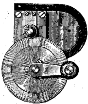
Рукоятка вызывнаго телефоннаго аппарата, при вращеніи которой возбуждается индукціонный токъ. См. текстъ, стр. 345.
