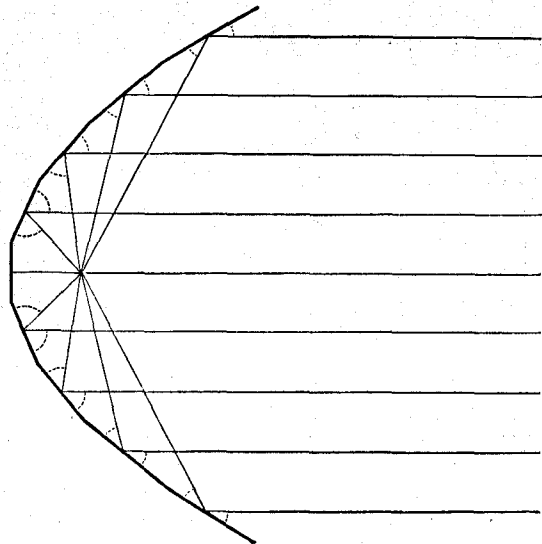
Отраженіе лучей въ системѣ плоскихъ зеркалъ, расположенныхъ по параболѣ. См. текстъ, стр. 197.
