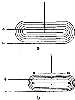
Положеніе магнитной стрѣлки въ мультипликаторѣ гальванометра. а простая стрѣлка, в аstaticкая стрѣлка. См. текстъ, стр. 330.
