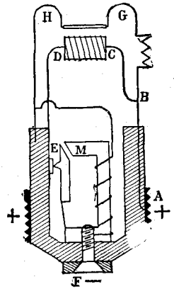
Схема устройства лампы Нерста съ электрическимъ нагрѣвателемъ. См. текстъ, стр. 324.
