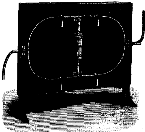
Гидравлическая модель Витстонова мостика. По Шписер-Эрнске. См. текстъ, стр. 323.
