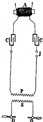
Схема полувольнаго тока Теслы. См. текстъ, стр. 352.
