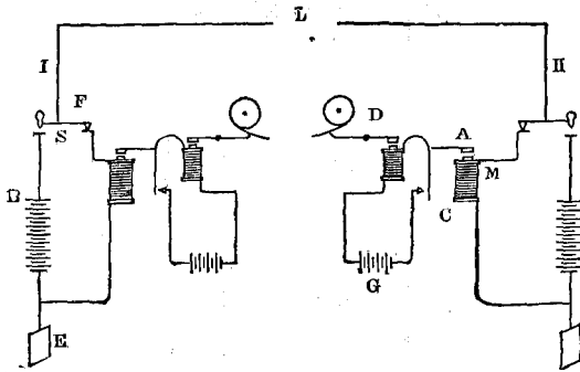
Схематическое изображение двухъ телеграфныхъ станцій. См. текстъ, стр. 334.
