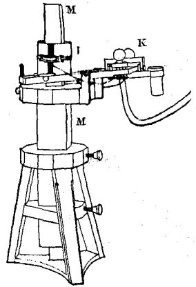
Гауссова станція отправки. См. текстъ, стр. 340.
