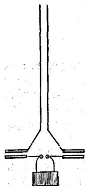
Опыты Герца. Доказательство независимости длины волны отъ материала проводниковъ. См. текстъ, стр. 362.
