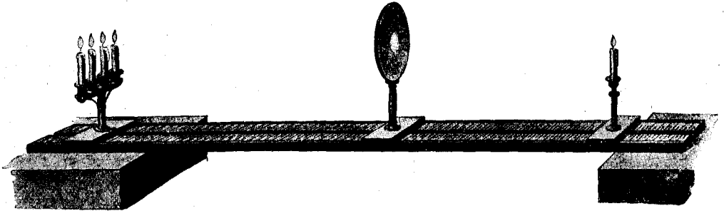
Фотометръ съ жирнымъ пятномъ, Бунзена. См. текстъ, стр. 193.
