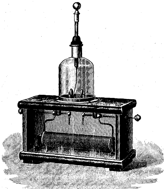
Дамоніевъ столбъ изъ листовъ сусальнаго золота и серебра, съ Фехнеровымъ электрометромъ. См. текстъ, стр. 317.
