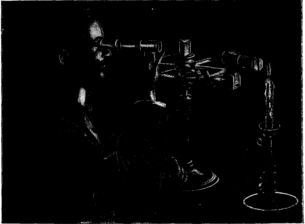
Отражательный-гонометръ. Измѣреніе угла призмы. См. текстъ, стр. 196.
