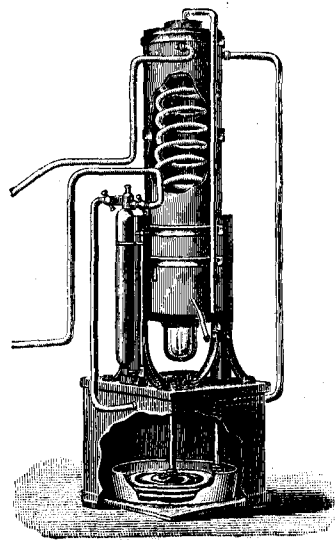
Машина Лиде. в. схематическое изображение.
