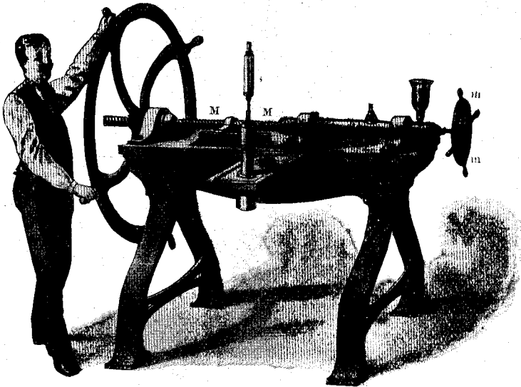
Приборъ Кальетэ для ожигенія постоянныхъ газовъ. См. текстъ, стр. 163.
