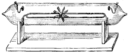
Катодная мельница. См. текстъ, стр. 376.
