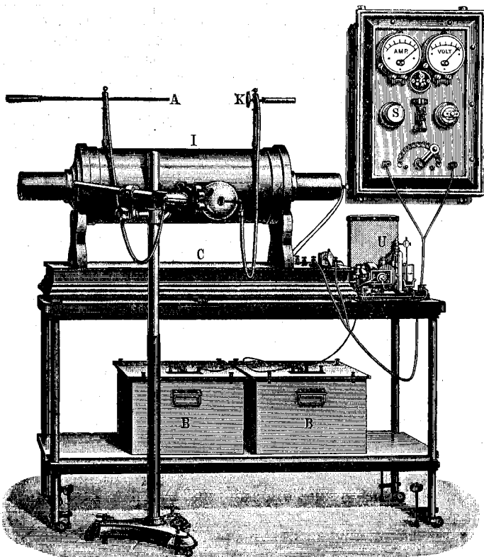
Приборъ для рентгенизаціи, возбуждаемый аккумуляторами. См. текстъ, стр. 390.
