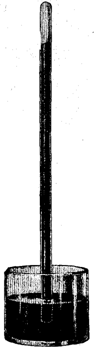
Ртутный столбъ, вогнанный въ трубку давленіемъ воздуха. См. текстъ, стр. 103.
