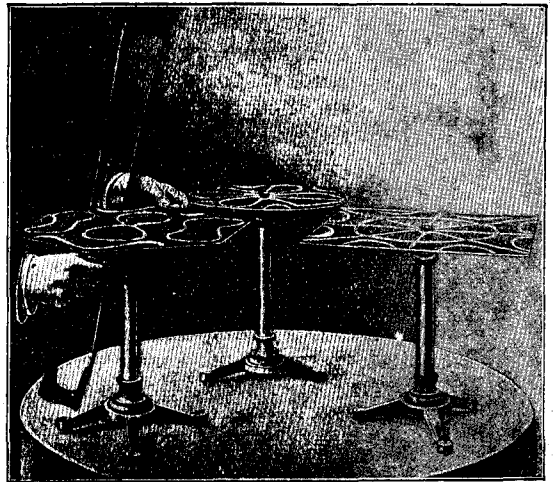
Хладниевы фигуры. См. текстъ, стр. 133.
