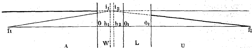
Схема глаза. См. текстъ, стр. 246.
