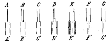
Цеемановское явленіе. См. текстъ, стр. 290.
