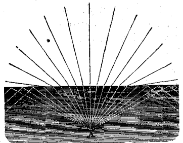
Полное внутреннее отраженіе См. текстъ, стр. 210.
