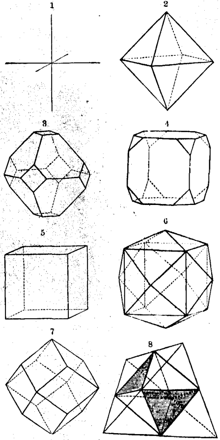
Простыя формы кристалловъ правильной системы. 1. Равныя и взаимноперпендикулярныя оси правильной системы. 2. Октаедръ. 3. Октаедръ съ срѣзанными углами. 4. Переходная форма (отъ октаедра къ кубу). 5. Кубъ. 6. Пирамидальный кубъ. 7. Ромбическій додекаедръ. 8. Иолученіе тетраедра изъ октаедра путемъ гемидри. См. текстъ рядомъ.
