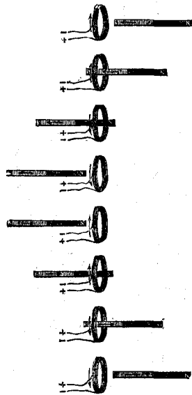
Направленіе наведеннаго тока по отношенію къ движенію магнита. См. текстъ, стр. 336.
