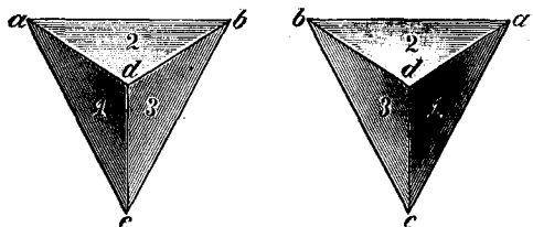
Два тетраэдра съ несимметричнымъ распределеніемъ поверхностей. См. текстъ рядомъ.
