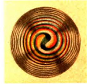
9. Кварцъ, спираль квадратной формы.
