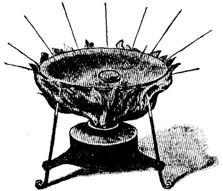
Явленіе Лейденфроста. См. текстъ, стр. 160
