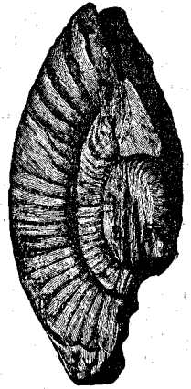
Аммонитъ, растянутый давлениемъ. Изъ „Періода бурь и натиска на земль“, Гаага. См. текстъ, стр. 113
