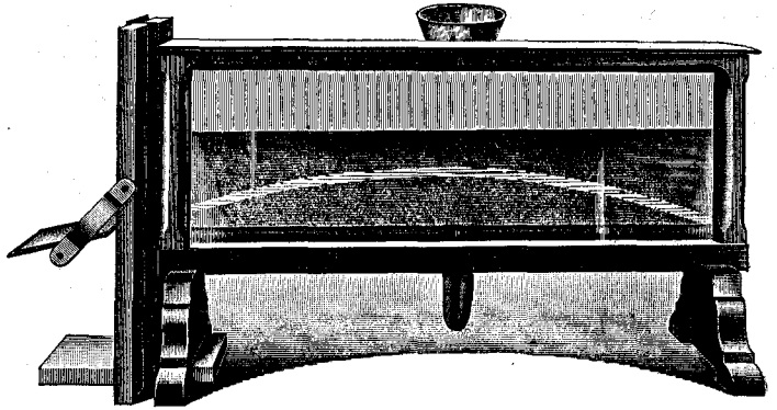
Преломленіе свѣта въ средахъ неодинаковой плотности. См. текстъ ниже.
