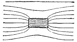
Сближеніе силовыхъ линий въ магнитѣ. См. текстъ, стр. 280.
