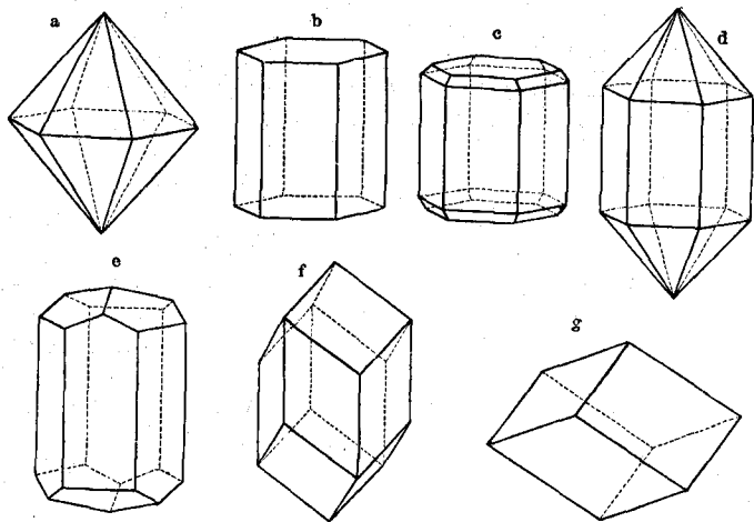
Гексагональная система.
