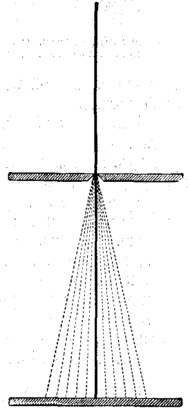
Диффракція свѣта, См. текстъ, стр. 258.
