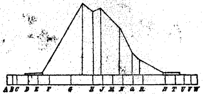
Кривая химическихъ дѣйствій свѣта въ разныхъ частяхъ свѣтового спектра. См. текстъ, стр. 274.
