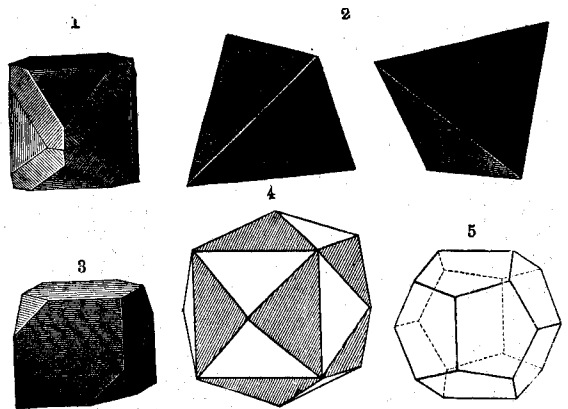
Переходъ кристалловъ правильной системы изъ одной формы въ другую. 1. Октаэдръ съ сръзанными углами. 2. Симметричные тетраэдры. 3. Соединеніе куба съ тетраэдромъ. 4. Превращеніе пирамидальнаго куба въ пентагональный додекаэдръ (путемъ возникновенія заштрихованныхъ на чертежѣ граней). 5. Пентагональный додекаэдръ. См. текстъ, стр. 488.
