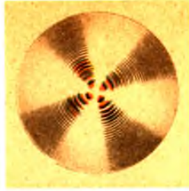
2. Известковый шпатель, бѣлый крестъ.
