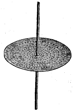
Силыныя линіи прямолинейнаго гальваническаго тока. См. текстъ, стр. 331.
