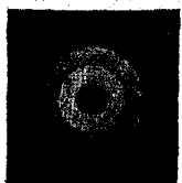
Строеніе пламени. См. текстъ стр. 441.
