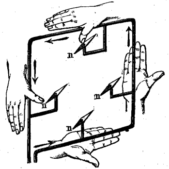
Правило Ампера. См. текстъ, стр. 331.
