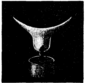
Дѣйствіе магнита на пламя. См. текстъ, выше.
