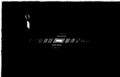
Явленіе диффракціи. О отверстіи, черезъ которое проходитъ свѣтъ. См. текстъ, стр. 258.
