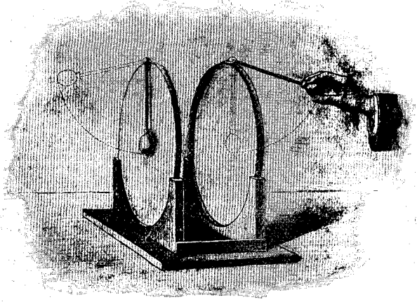
Передача удара воздухомъ. См. текстъ, стр. 121.
