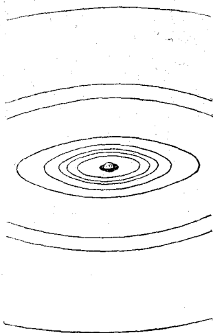
Орбиты спутниковъ Сатурна.
