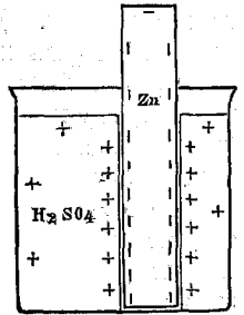
Раздѣленіе электричества въ электролитахъ. См. текстъ, стр. 560.
