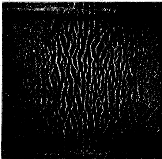
Фигуры Декартова на пескѣ. Изъ „Archive des séances physiques, Genève“. См. текстъ, стр. 89.
