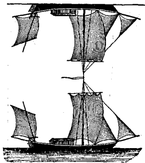
Миражъ, наблюдаемый на морѣ. См. текстъ, стр. 206.
