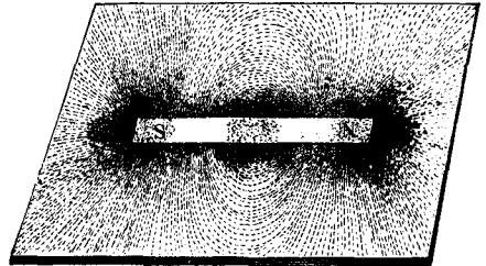
Распределение желѣзныхъ опилокъ вокругъ магнита. N сѣверный полюсъ, S южный полюсъ. См. текстъ, стр. 278.
