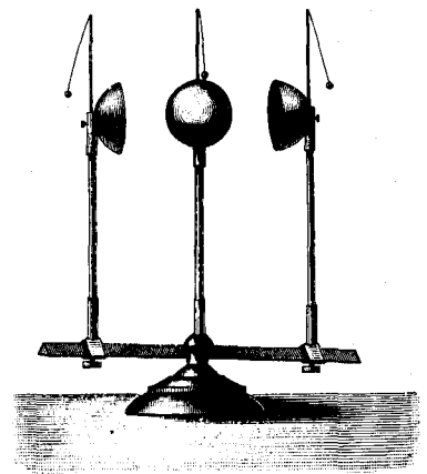
Распространеніе электричества по поверхности. См. текстъ выше.
