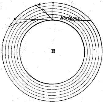
Рефракція, или лучепреломленіе въ атмосферѣ. Кажущееся положеніе звѣзды. Истинное положеніе звѣзды; E — земля. См. текстъ, стр. 205.
