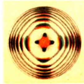
8. Кварцъ, кольца въ видѣ квадратовъ.
