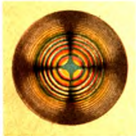
7. Кварцъ, круговыя кольца.
