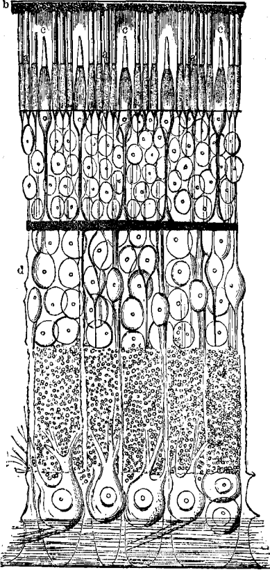
Палочки и колбочки въ сѣтчаткѣ. а) Палочки; б) Пигментный слой; в) Колбочки; г) Нервн. клѣтки. См. текстъ, стр. 250.
