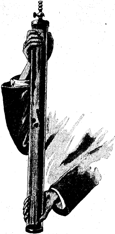
Паденіе тѣлъ въ безвоздушномъ пространствѣ.
