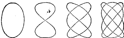
Фигуры Лиссажу. См. текстъ, стр. 136.
