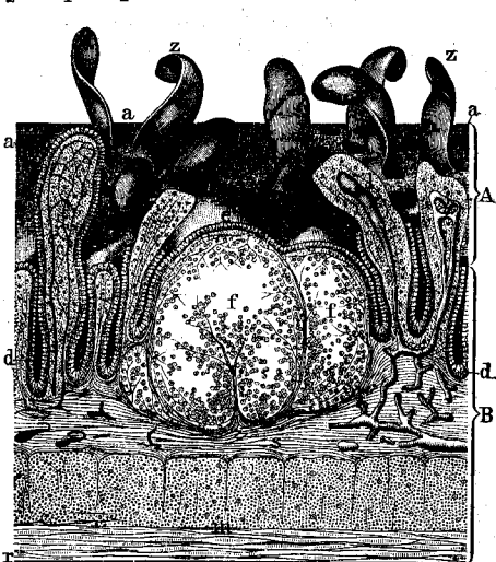
Разрѣзъ слизистой оболочки тонкой кишки. z Ворсинки, с кровоносные сосуды, лимфатические сосуды, а отверстие железъ, m мышечная ткань, f млечные сосуды. См. текстъ, стр. 595.
