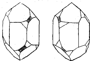
Кристаллы кварца. См. текстъ рядомъ.
