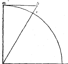
Движеніе тѣла по инерціи въ то же время подь влияніемъ силы притяженія.
