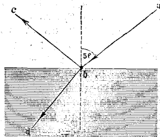
Уголъ наибольшей поляризаціи. См. текстъ выше.
