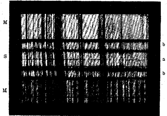
Спектръ Сатурна между лунными спектрами. S спектръ Сатурна (a спектръ ядра, bb спектръ кольца), MM лунный спектръ. См. текстъ, стр. 240.
