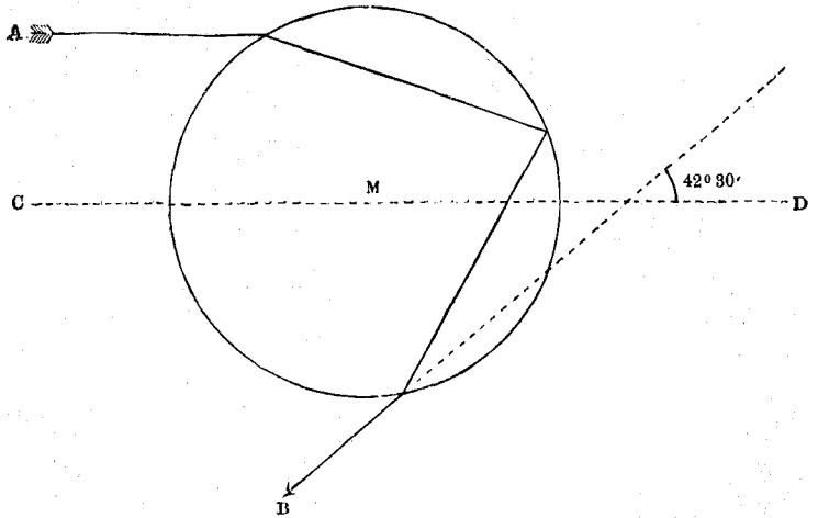
Ходъ свѣтового луча въ каплѣ воды при образованіи радуги. А Свѣтовой лучъ, попадающій въ каплю воды М въ моментъ нахождения солнца на горизонтѣ, В лучъ красного цвѣта, выходящій изъ капли, составляющій съ горизонтомъ уголъ 42^{\circ} 30' , CD горизонтъ.
