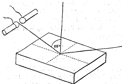
Поляризація электрическихъ лучей. См. текстъ, стр. 361.
