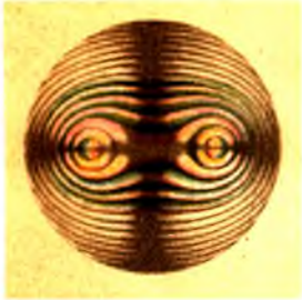
4. Селитра, черный крестъ.
