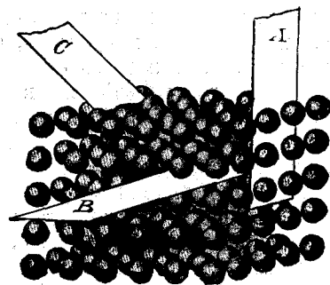
Схема сопротивлений кристалла кубическаго строения при паденіи на него свѣтовыхъ лучей по различнымъ направленіямъ. См. текстъ, стр. 266.
