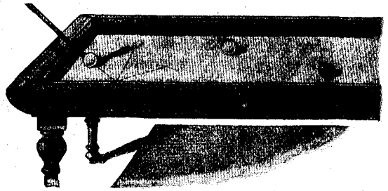
Отраженіе бильярднаго шара. См. текстъ, стр. 90.
