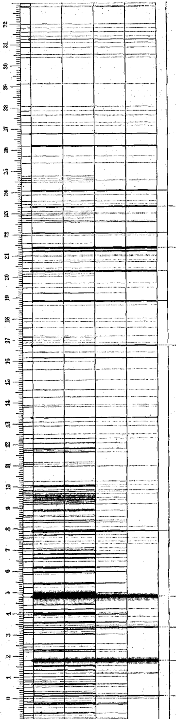
Часть солнечнаго спектра Толлона, смежная съ двойной линіей натрія. См. текстъ, стр. 238. Титанъ. Натрій. Натрій. Натрій. Натрій. Титанъ. Каллистъ. Барій.
