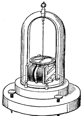
Гальванометръ съ аstaticкой стрѣлкой. См. текстъ, стр. 330.
