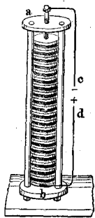
Вольтовъ столбъ, состоящій изъ паръ цинковыхъ и мѣдныхъ пластинокъ, съ прокладками изъ влажной бумаги. См. текстъ, стр. 317.
