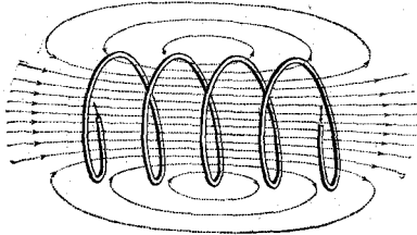
Силыяя линіи гальванической спирали. См. текстъ, стр. 332.
