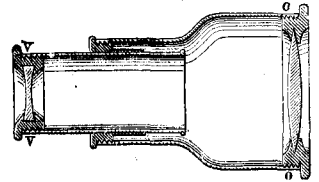
Бинокль. См. текстъ, стр. 216.
