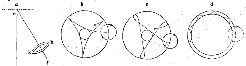
а ось волчка; б, с, d кривыя, описываемыя концомъ волчка. См. текстъ, стр. 85.
