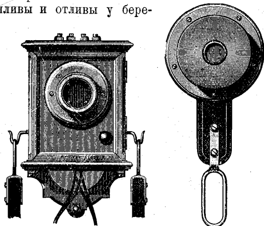
Телефонный аппаратъ, съ висащими на немъ телефонными трубками, имѣющіяся въ управленіи имперскихъ телефоновъ (Германія). в. Трубка. См. текстъ, стр. 342.
