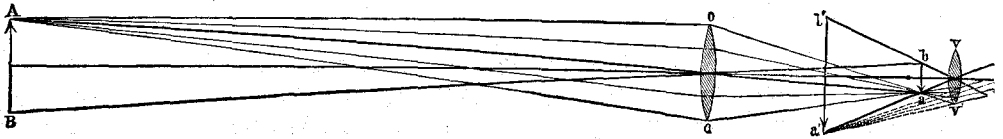
Подзорная труба Кеплера. См. текстъ, стр. 215.
