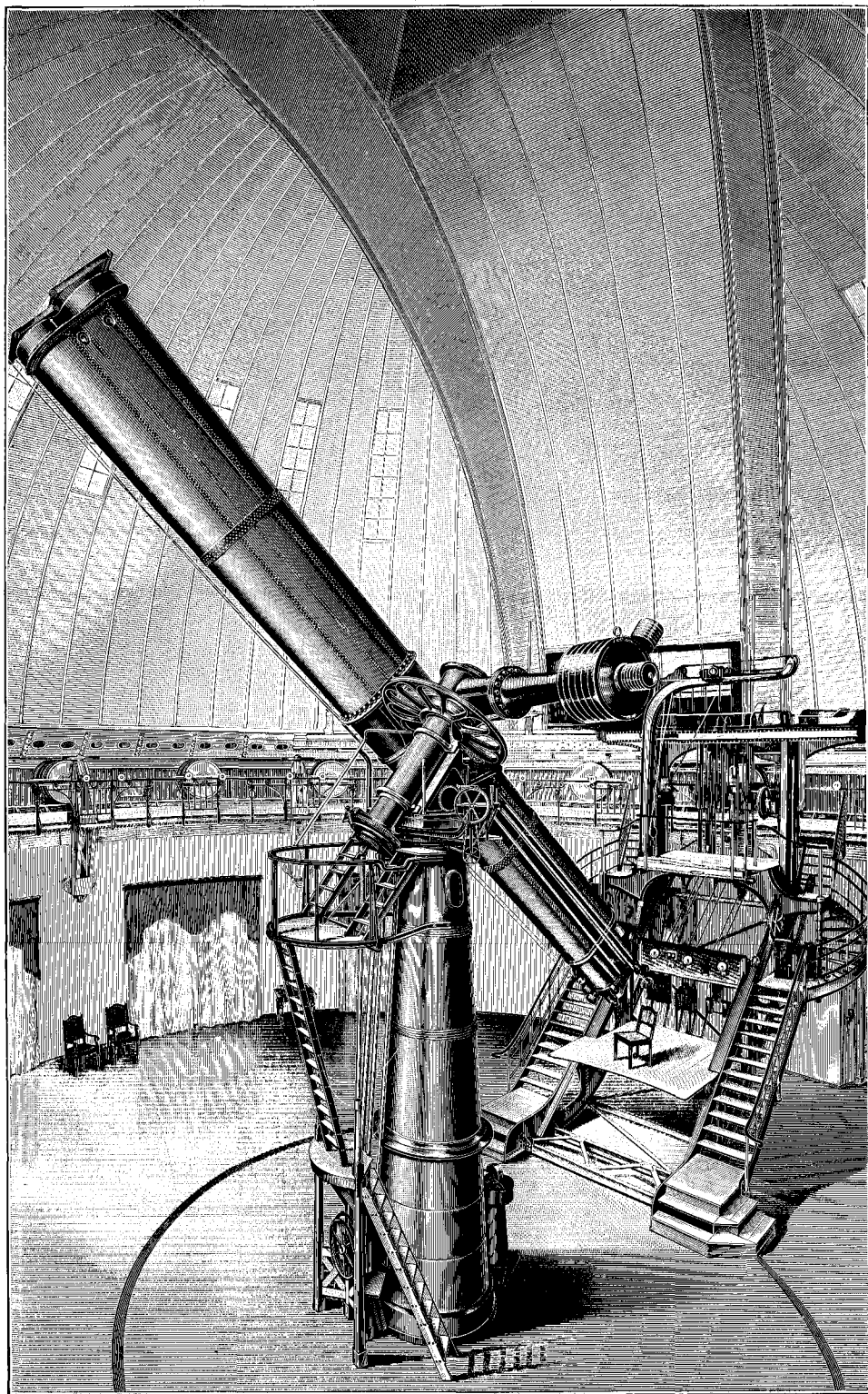
Большой рефракторъ астрофизической обсерватори въ Потсдамѣ.
