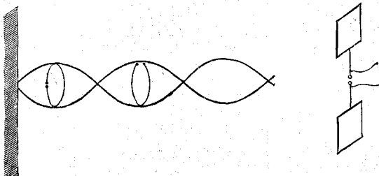
Измѣреніе длины свѣтовыхъ волнъ при помощи резонатора Герца. См. текстъ, стр. 360.
