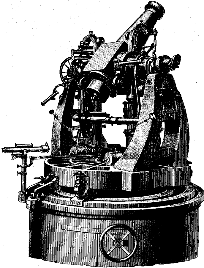
Ломаная труба (альтазимуть). См. текстъ, стр. 217.
