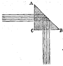
Призма полного внутреннего отраженія. См. текстъ, стр. 211.
