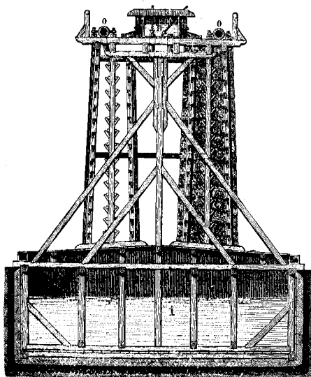
Разрѣзъ градирни. o, n трубы; h кладка тростника; i резервуаръ. См. текстъ, стр. 431.
