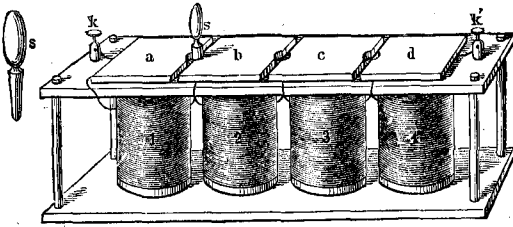
Реостатъ съ штепселями по Сименсу, вѣдъ сопротивленія; s штепель; 1—4 катушки сопротивленій. См. текстъ, стр. 322.
