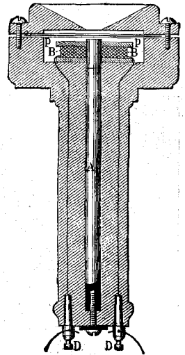
Разрѣзъ телефонной трубки Белла. См. текстъ, стр. 342.
