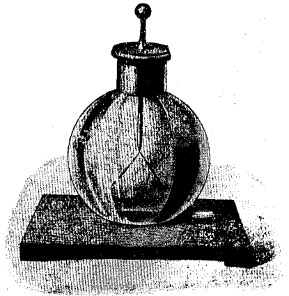
Электроскопъ съ золотыми листочками. См. текстъ ниже.
