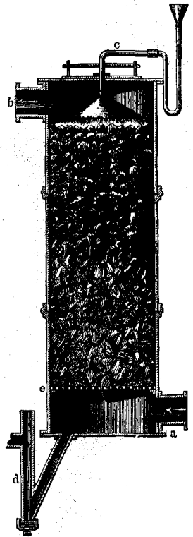
Коксовый цилиндръ для промыванія свѣтильнаго газа. См. текстъ, стр. 459.
