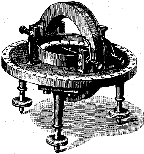
Тангенсъ-гальванометръ. По Сименсу и Гальсѣ. См. текстъ, стр. 331.
