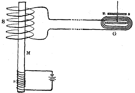
Индукціонный токъ. См. текстъ, стр. 337.
