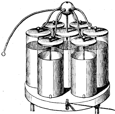
Батарея Рисса, составъ изъ лейденскихъ банокъ. См. текстъ, стр. 309.
