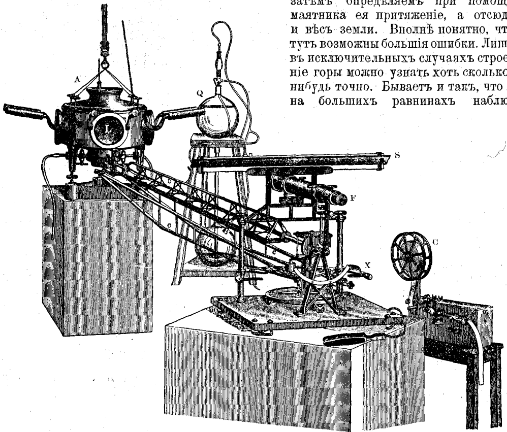
Точные вѣсы Вунге въ международномъ бюро мѣръ. („Bureau international des poids et des mesures“, Guillaumet). См. текстъ, стр. 63. А. мѣсто, гдѣ находятся самыя вѣсы. L. окно, черезъ которое наблюдается наклонъ коромысла помощью зрительной трубы F. S. скала, на которую отбрасывается свѣтовое пятно. C. хронографъ для электрической записи движеній свѣтового пятна. X. ручка для накладыванія на чашки грузовъ. Q. ртутный насосъ, служащій для выкачиванія воздуха изъ А.
