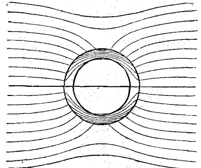
Полый желѣзанный шаръ въ однородномъ магнитномъ полѣ. См. текстъ, стр. 351.
