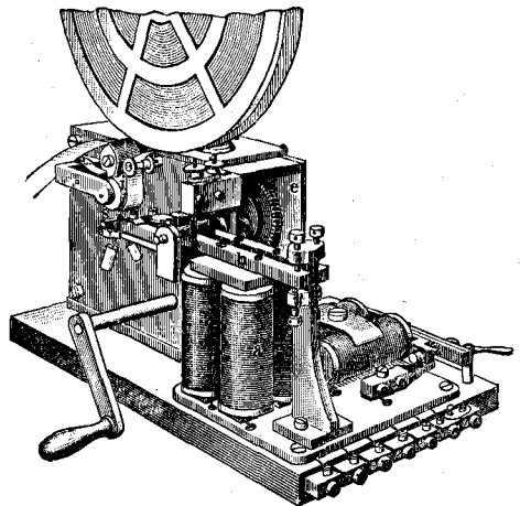
Электрический хронографъ Фюса. См. текстъ, стр. 335.
