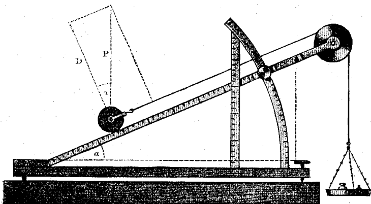
Разложеніе силъ на наклонной плоскости. См. текстъ, стр. 78.
