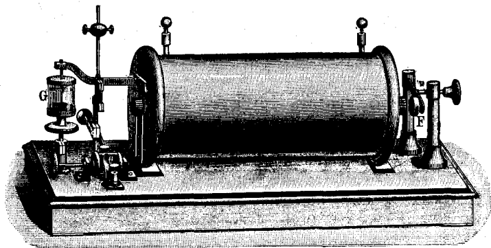
Небольшая индукціонная спираль съ ртутнымъ прерывателемъ и Вагнеровскимъ молоточкомъ. См. текстъ, стр. 387.
