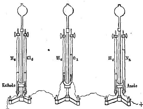
Опредѣленіе отношенія числа атомовъ веществъ, образующихъ молекулу, при помощи разложенія въ voltaметрахъ. Voltaметры съ а) соляной кислотой б) водой в) аммиакомъ. См. текстъ, стр. 506.
