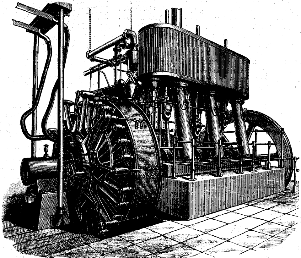
Машина постоянного тока Сименсъ и Гальске. См. текстъ, стр. 352.
