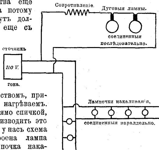
Схема расположения проводов электрического освѣщенія. См. текстъ, стр. 323.
