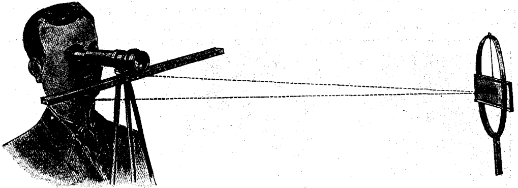
Зеркальный отсчетъ. См. текстъ, стр. 195.
