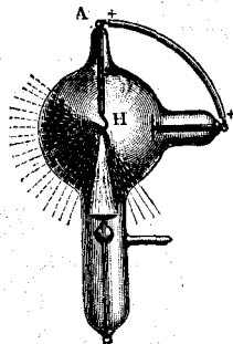
Рентгеновская трубка съ вогнутымъ платиновымъ зеркаломъ въ фокусѣ катодныхъ лучей. См. текстъ ниже.
