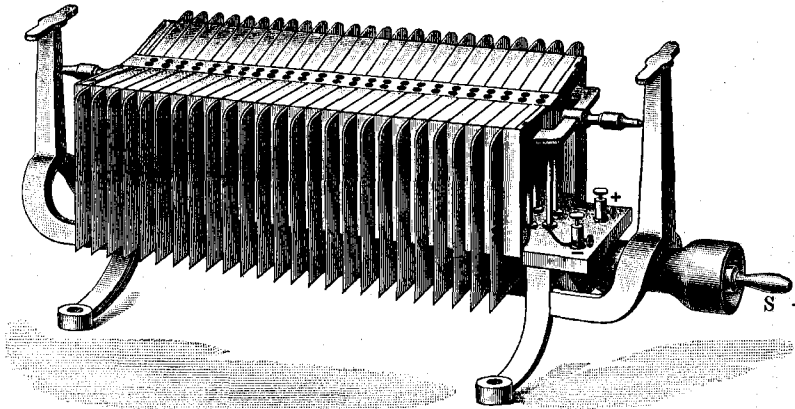
Термоэлектрическій столбъ. См. текстъ, стр. 368.
