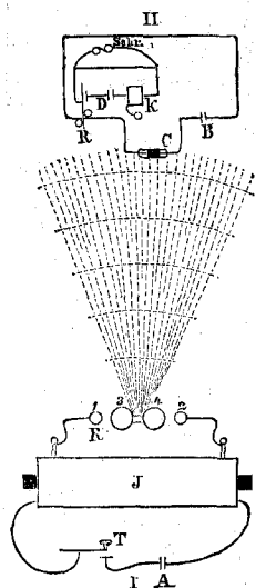
Принципъ беспроволочнаго телеграфированія. См. текстъ, стр. 366.
