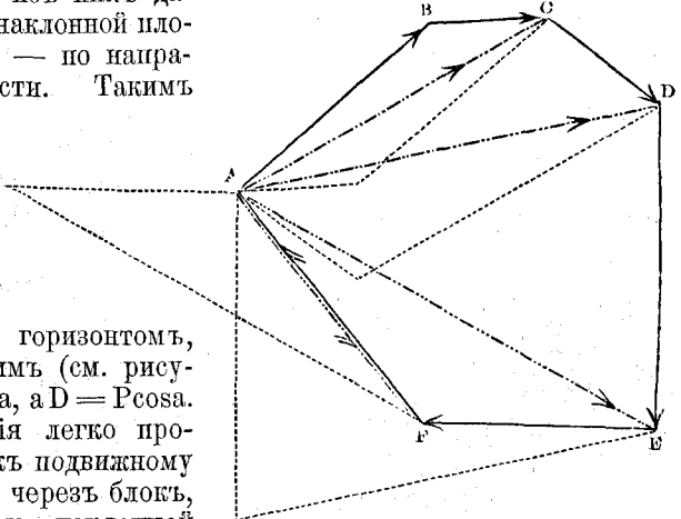
Статическій многоугольникъ. Случай тѣла, испытывающаго дѣйствіе нѣсколькихъ силъ сразу. См. текстъ, стр. 76.
