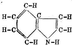
Индолъ C 8 H 7 N
