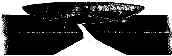
Дѣйствіе магнита на жидкость. См. текстъ, стр. 289
