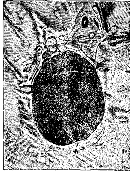
Цѣрки на лунѣ: а) при восходѣ солнца б) въ полдень. Изъ „Мірозданія“, В. Мейера. См. текстъ ниже.
