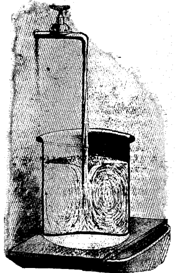
Вихрь въ водѣ. См. текстъ, стр. 281.
