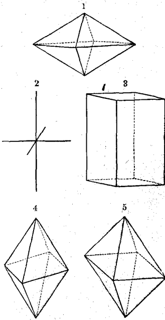
Кристаллы ромбической, моноклинической (одноклиномѣрной) и триклинической (трехклиномѣрной) системы. 1. Пирамида ромбической системы. 2. Расположеніе осей въ кристаллахъ ромбической системы. 3. Призма ромбической системы. 4. Випирамида одноклиномѣрной системы. 5. Випирамида трехклиномѣрной системы. См. текстъ, стр. 491.
