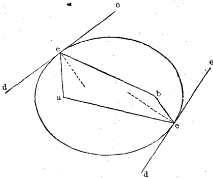
Отраженіе звука въ эллипсѣ. См. текстъ, стр. 128.
