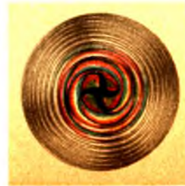
11. Кварцъ, спираль Эйри.
