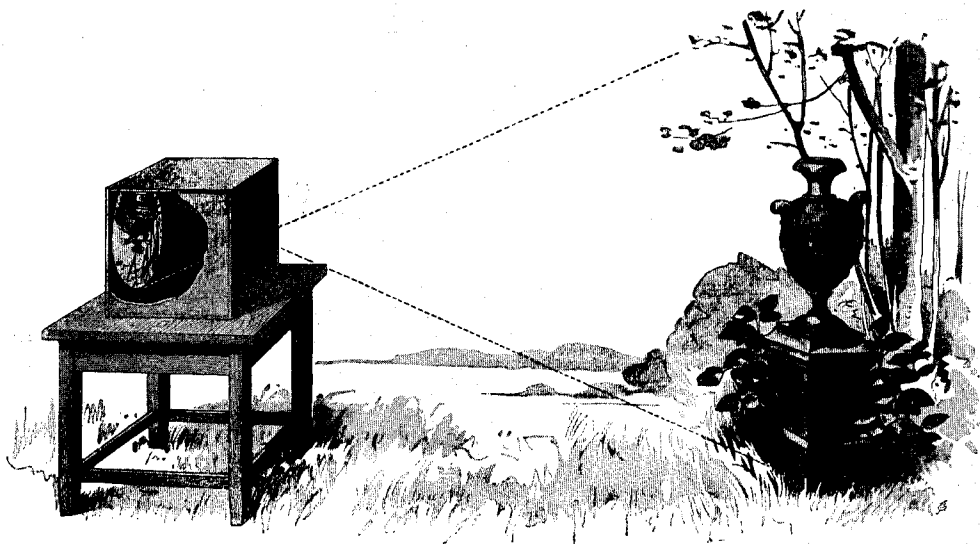
Полученіе изображенія въ камерѣ-обскурѣ съ простымъ отверстиемъ. См. текстъ, стр. 190.
