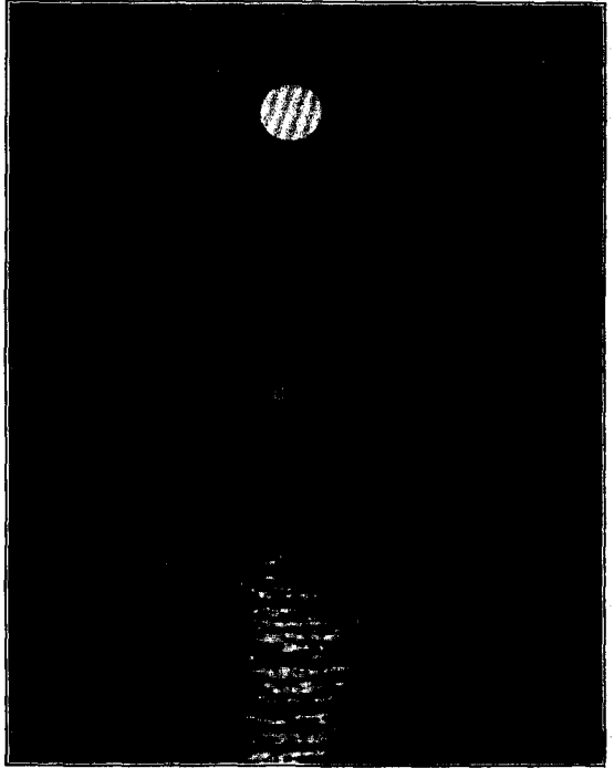
Эллиптическая форма солнечнаго диска, какъ результатъ лучепреломленія. Моментальный снимокъ съ латуры. См. текстъ, стр. 203.
