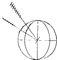
Обыкновенный лучъ (а) и необыкновенный лучъ (б) въ положительномъ одноосномъ кристаллѣ. См. текстъ ниже.
