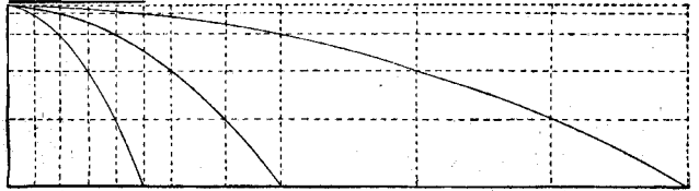
Параболы, описываемыя падающими тѣлами. См. текстъ стр. 52.
