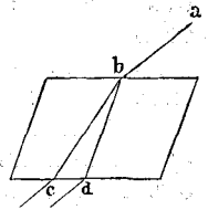
Лучи обыкновенный и необыкновенный въ исландскомъ шпатѣ. См. текстъ, стр. 269.
