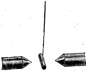
Положеніе діамагнитнаго висмута между полюсами магнита. См. текстъ, ниже.
