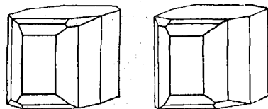
Асимметричныя кристаллы винной кислоты. См. текстъ, стр. 462.
