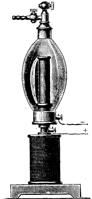
Искусственное полярное сіаніе въ Гейсслеровой трубкѣ См. текстъ, стр. 380.
