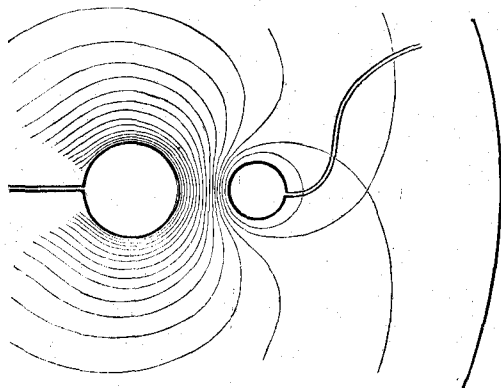
Линіи равнаго потенциала. См. текстъ, стр. 307.
