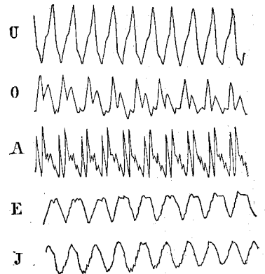
Фонографическія записи пяти гласныхъ, пропѣтыхъ на ноту одной и той же высоты. См. текстъ выше.
