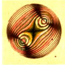
5. Селитра, гиперболы.
