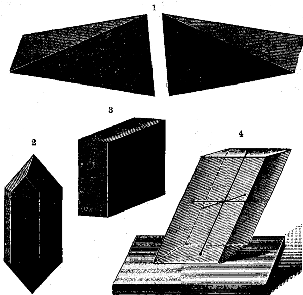
1. Тетраедръ ромбической системы. 2. Столбчатый шестиугольный кристаллъ ромбической системы. 3. Призма однонаклонной системы. 4. Призма трехнаклонной системы. См. текстъ, стр. 490.
