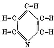
Пиридинъ C 5 H 5 N
