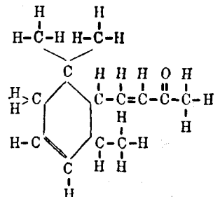
Соединеніе, обуславливающее запахъ фіалокъ \text{C}_{15}\text{H}_{20}\text{O} .
