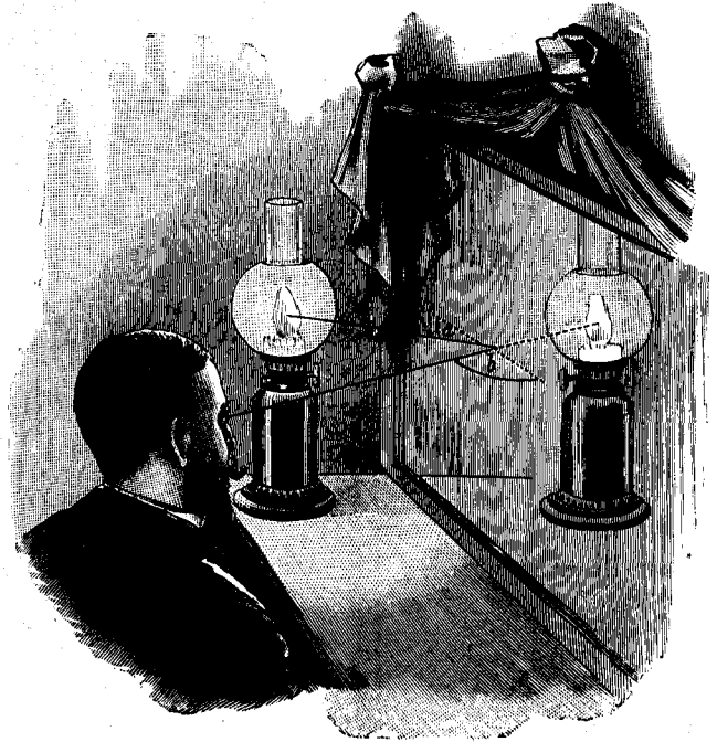
Отраженіе свѣта въ плоскихъ зеркалахъ. Изъ „Мирозданія“, В. Мейера. См. текстъ, стр. 194.
