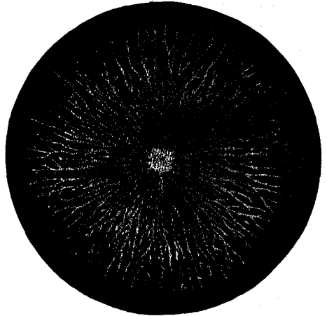
Лихтенберговы фигуры. См. текстъ, стр. 312.
