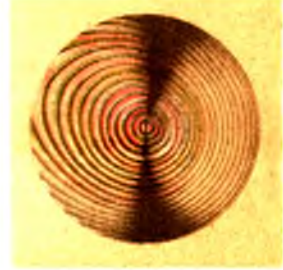
6. Сахаръ, круговыя кольца не имѣютъ правильной формы.
