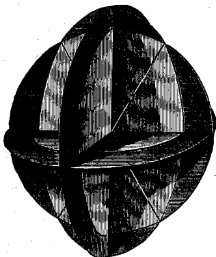
Поверхность волны въ кристаллахъ системъ ромбической, одноклиномѣрной и трехклиномѣрной. См. текстъ выше.
