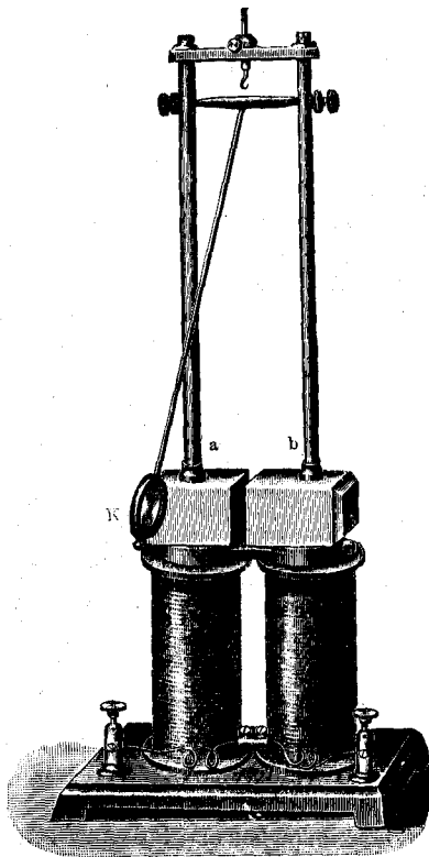
Маятникъ Вальтенгофена. См. текстъ, стр. 339.
