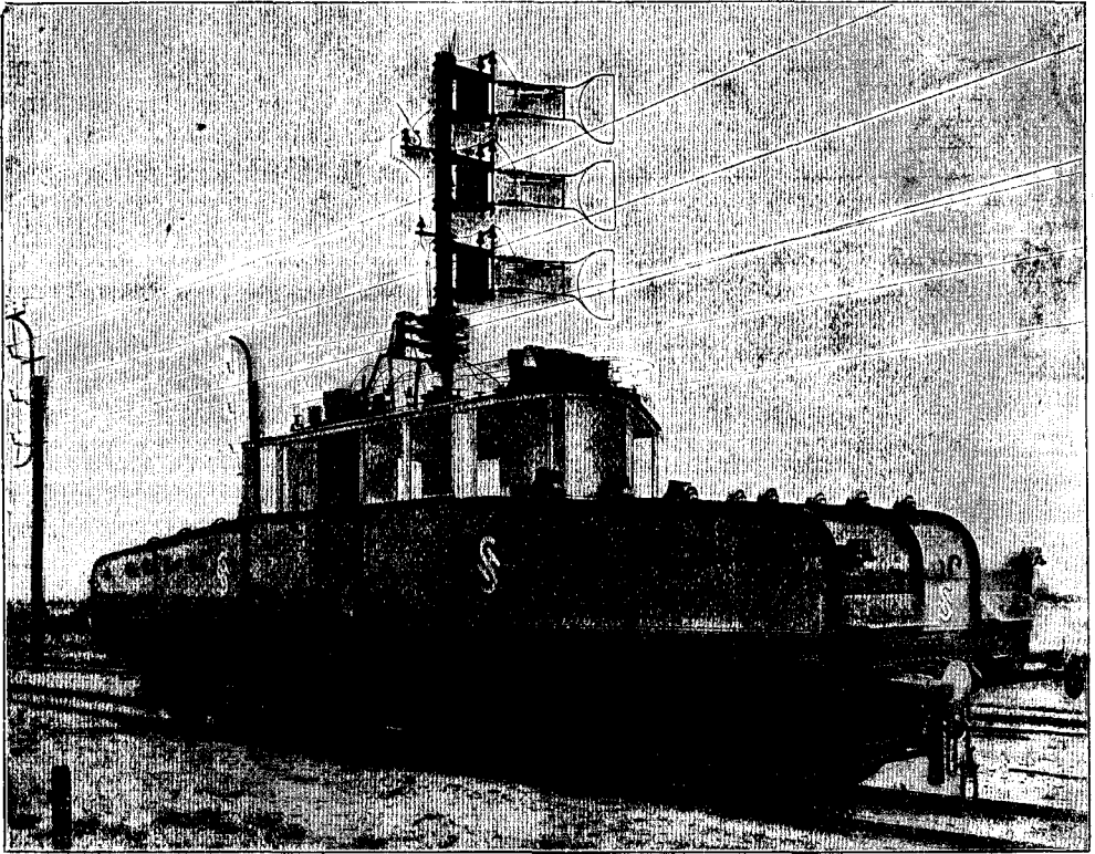
Выстроходный электровозъ системы Сименса и Гальске. См. текстъ, стр. 349.
