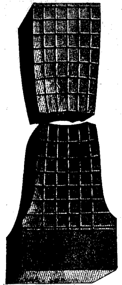
Пластичность желѣза при растяженіи. См. текстъ, стр. 113.
