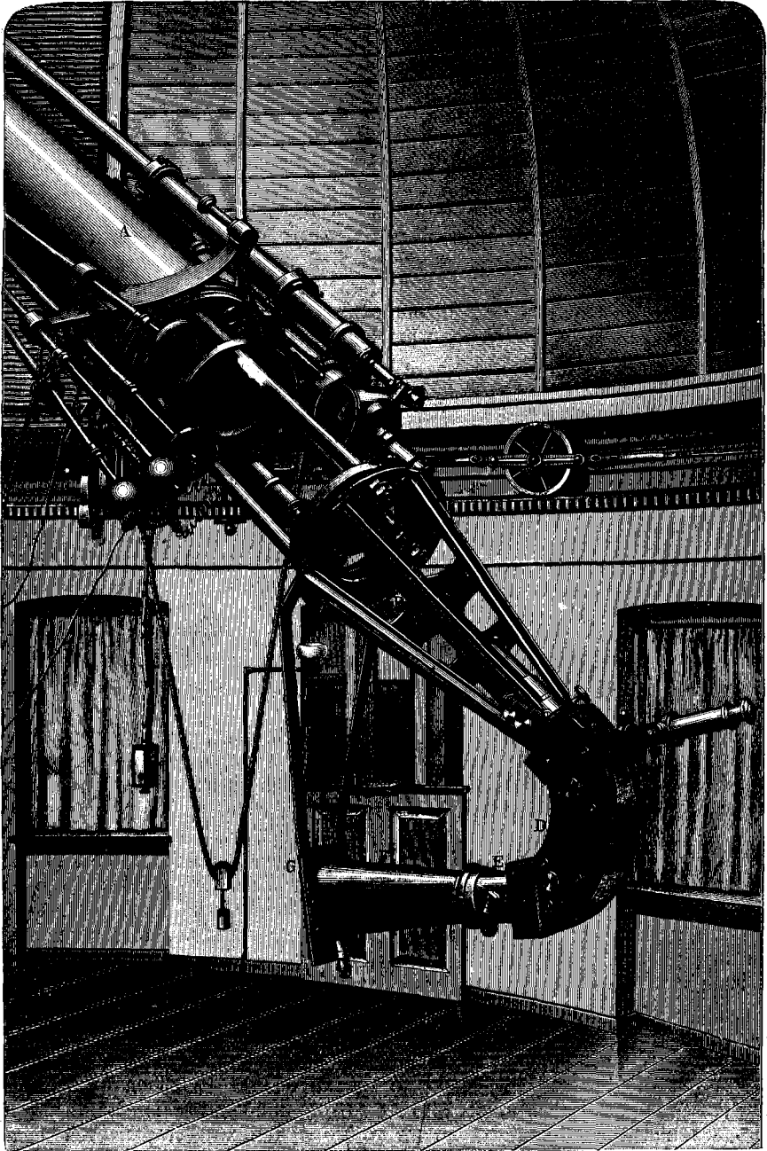
Спектрографъ астрофизической обсерваторіи въ Потсдамѣ. Свѣтовые лучи черезъ объективъ рефрактора A проходятъ въ коллиматоръ BC ; отсюда черезъ щель, находящуюся въ C , они переходятъ въ линію D ; отразившись тамъ отъ помѣщенныхъ въ немъ призмъ, поступаютъ въ фотографическую камеру EF и кассетту G , гдѣ и фиксируются на свѣточувствительной пластинкѣ. См. текстъ, стр. 239.
