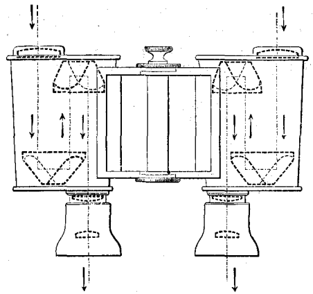
Разрѣзъ двойной трубы Гейсса. См. текстъ, стр. 217.
