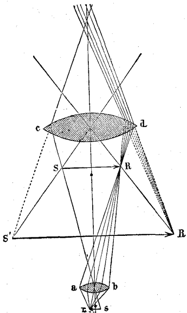
Ходъ лучей въ сложномъ микроскопѣ: га предметъ; ab объективъ; cd окуляръ; SR действительное изображение; S, R, увеличенное изображение. См. текстъ, стр. 217.
