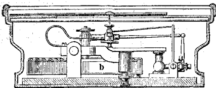
Поперечное сѣченіе.
