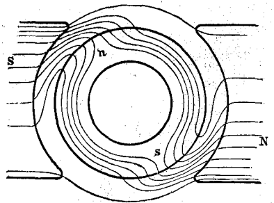
Линіи равнаго потенціала въ кольцѣ Пачинотти. См. текстъ, стр. 351.
