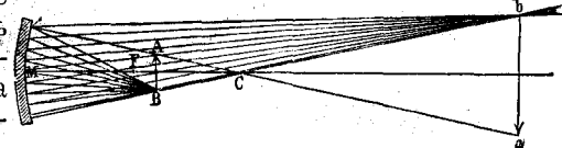
Дѣйствительное изображеніе въ вогнутомъ зеркалѣ. См. текстъ выше.
