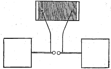
Вибраторъ Герца. См. текстъ, стр. 360
