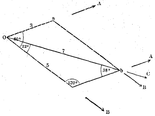
Построеніе параллелограмма силъ. См. текстъ, стр. 74.
