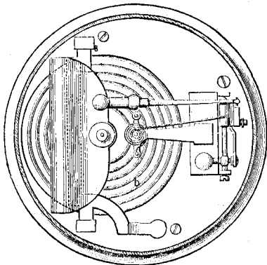
Общій чертежъ.
