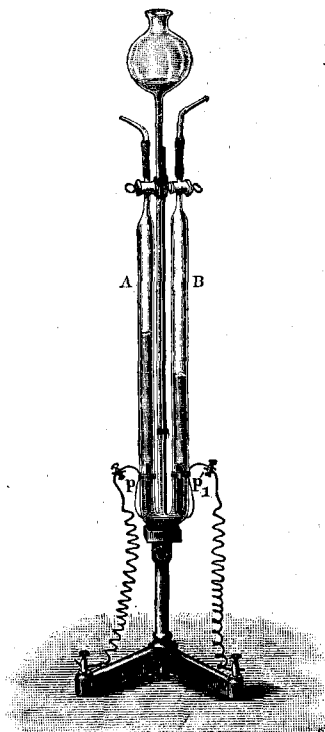
Разложение жидкости в вольтаметре. См. текст, стр. 370.
