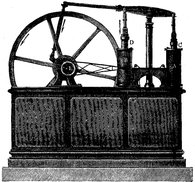
Электромагнитная машина Пелжа. DC магниты; AB катушкимультипликаторы; L маховое колесо. См. текстъ, стр. 334.
