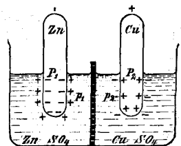
Возникновеніе электрическаго напряженія въ электролитахъ при погруженіи въ нихъ неодинаковыхъ металловъ. См. текстъ выше.
