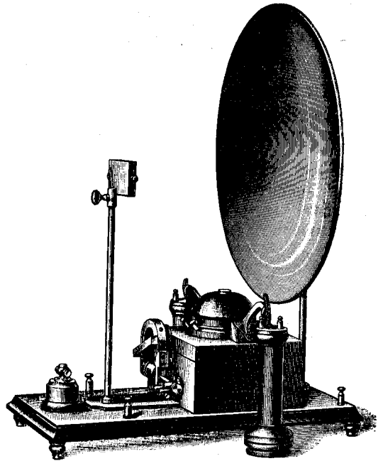
Селеновый столбикъ, какъ приемникъ при фонофонической передачѣ. См. текстъ, стр. 330.
