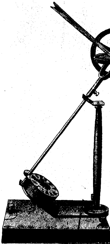
Гелиостатъ. См. текстъ ниже.
