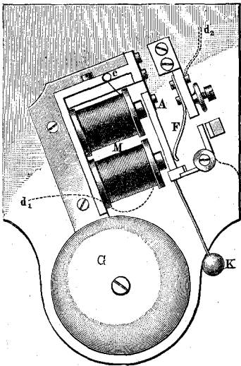
Телефонный звонокъ. См. текстъ, стр. 344.
