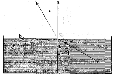
Лучепреломленіе. См. текстъ, стр. 210. а перпендикуляръ, возставленный въ точкѣ паденія; b лучъ, идущій по поверхности; сс лучъ, испытывающій полное внутреннее отраженіе; d предѣльный уголъ полного внутренняго отраженія.
