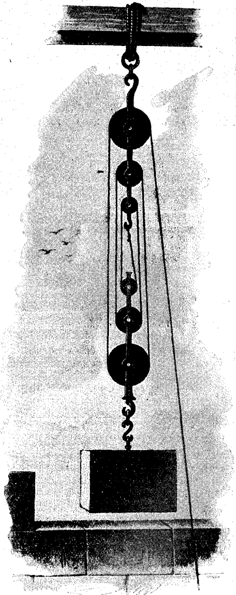
Полиспастъ. См. текстъ, стр. 71.
