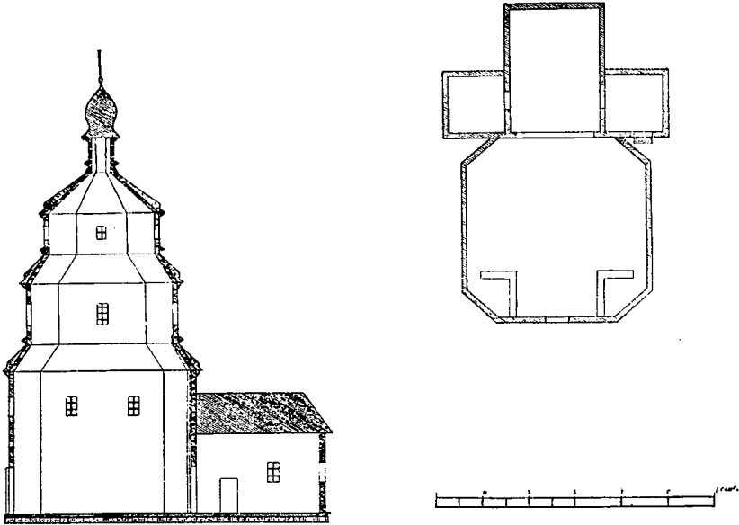
2. Церква в м. Торговиці, розріз, плян (масштаб в сажнях).
