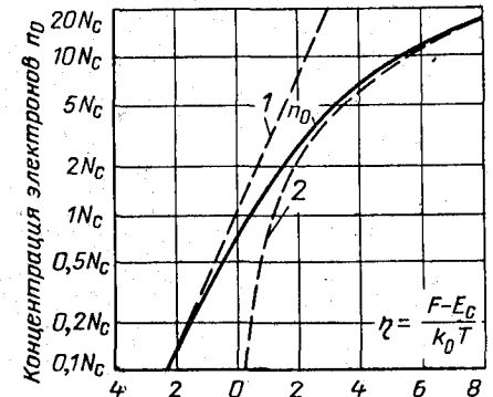
Рис. 3-3. Зависимость концентрации электронов проводимости от положения приведенного уровня Ферми.
