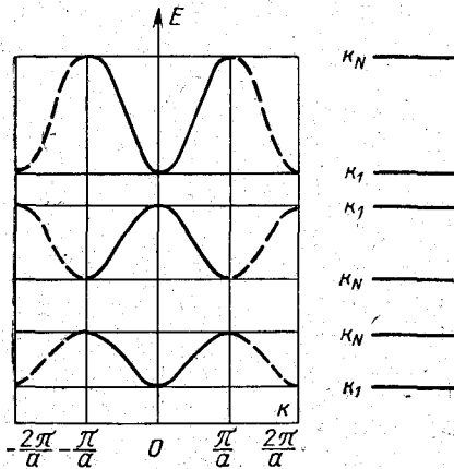
Рис. 2-9. Схематическая зависимость E(\kappa) для одномерной решетки в приближении сильно связанных электронов.
