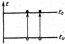
Рис. 3-5. Тепловая генерация носителей заряда в собственном полупроводнике.
