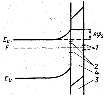
Рис. 9-7. Быстрые и медленные состояния на поверхности германия. 1 — медленные или внешние поверхностные состояния; 2 — быстрые или внутренние поверхностные состояния; 3 — слой окиси германия; 4 — запрещенная зона окиси.
