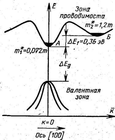
Рис. 5-8. Структура зон арсенида галлия в направлении оси [100].
