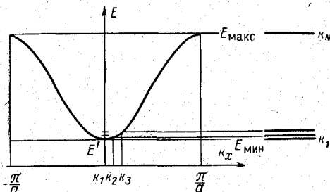
Рис. 2-6. Зависимость E(k_x) для s -состояния.
