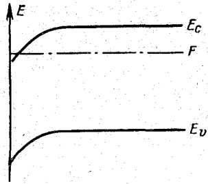
Рис. 9-2. Энергетическая диаграмма приповерхностной области полупроводника n -типа в случае обогащения.
