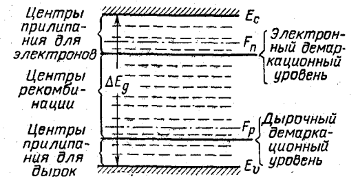
Рис. 6-9. Полупроводник, содержащий центры прилипания и центры рекомбинации.
