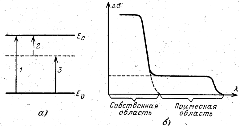
Рис. 11-9. Схематическое изображение переходов (а) и спектрального распределения фотопроводимости (б).
