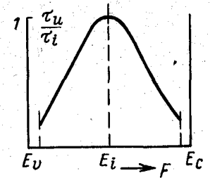
Рис. 6-5. Время жизни при ударной межзонной рекомбинации в зависимости от положения уровня Ферми.
