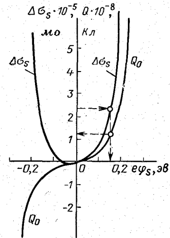
Рис. 9-5. Теоретические кривые поверхностной проводимости \Delta\sigma_s и плотности приповерхностного заряда Q_0 в зависимости от высоты барьера e\varphi_s для германия при комнатной температуре ( N_a = 3,4 \cdot 10^{13} \text{ см}^{-3} ).
