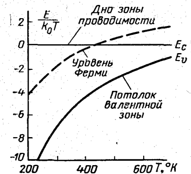
Рис. 3-9. Положение уровня Ферми (в единицах k_0 T ) в зависимости от температуры для антимонида индия.
