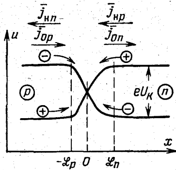
Рис. 8-13. Потенциальные барьеры для дырок и электронов в p - n переходе.
