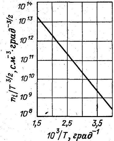
Рис. 3-7. Температурная зависимость n_i/T^{3/2} для германия.
