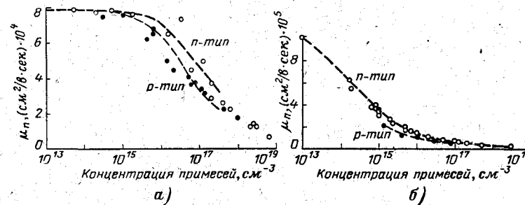
Рис. 5-1. Зависимость дрейфовой подвижности электронов от концентрации примесей в образцах антимонида индия n- и p-типа при 300° К (а) и 77° К (б). Пунктирные кривые — рассчитанные теоретически.
