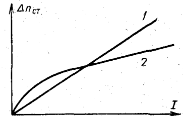
Рис. 11-6. Зависимость стационарной неравновесной концентрации электронов от интенсивности освещения для случая линейной (1) и квадратичной (2) рекомбинации.
