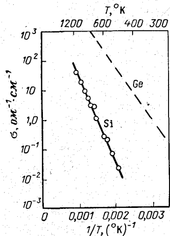
Рис. 1-3. Температурная зависимость удельной проводимости полупроводника.
