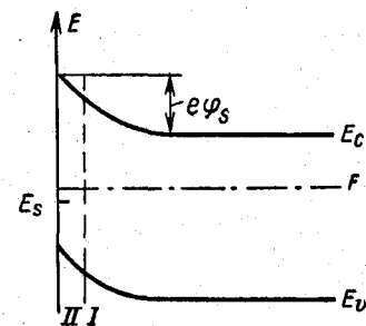
Рис. 9-1. Энергетическая диаграмма приповерхностной области полупроводника n-типа. I — область обеднения; II — область инверсии.
