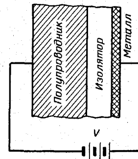
Рис. 9-4. Принцип измерения поверхностной проводимости при эффекте поля.
