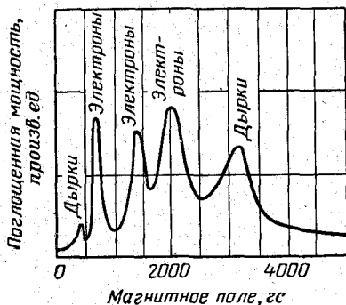
Рис. 2-14. Поглощение при циклотронном резонансе в германии.
