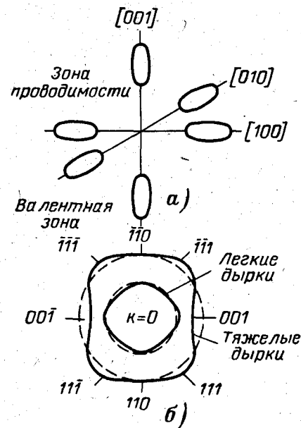
Рис. 2-18. Изоэнергетические поверхности в кремнии.
