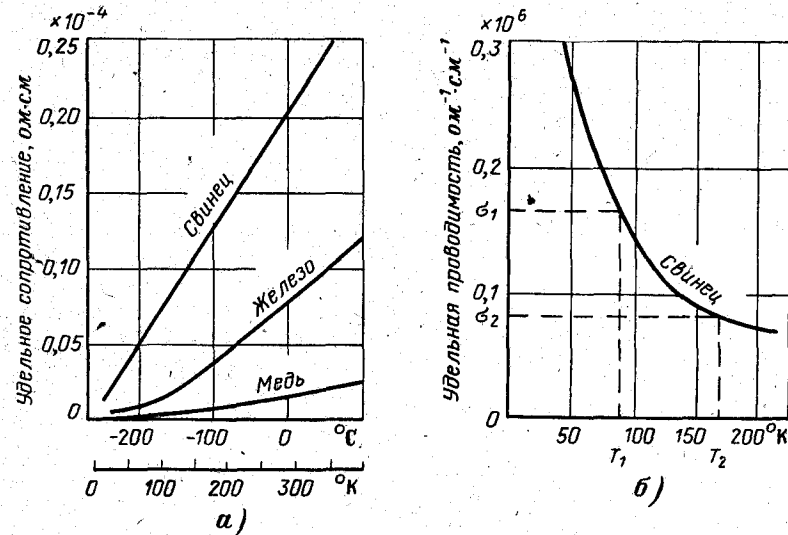
Рис. 1-2. Изменение удельного сопротивления чистых металлов (а) и удельной проводимости свинца (б) в зависимости от температуры.
