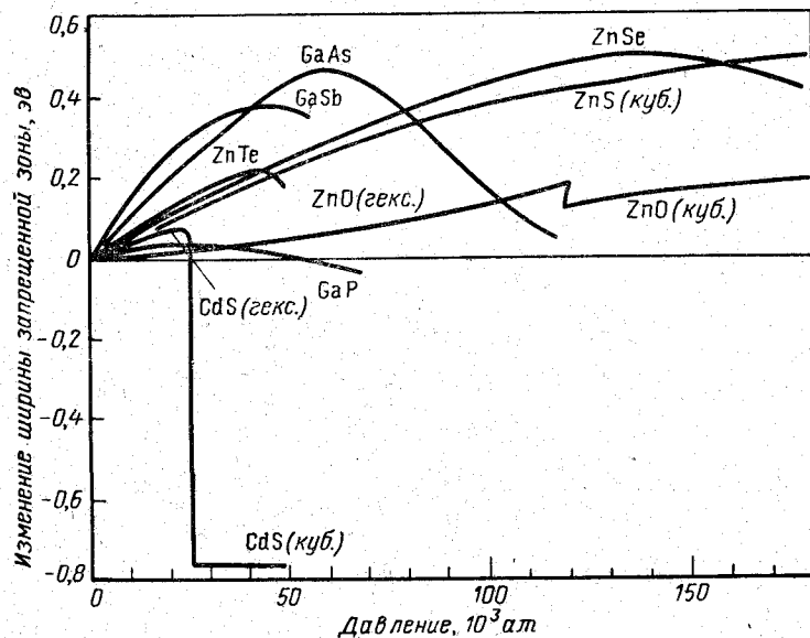
Рис. 10-17. Зависимость ширины запрещенной зоны от давления для некоторых полупроводников.
