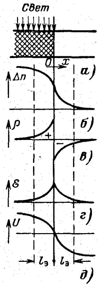
Рис. 7-3. Распределение концентрации (б), объемного заряда (в), электрического поля (г), потенциала (д) при частичном освещении донорного полупроводника.
