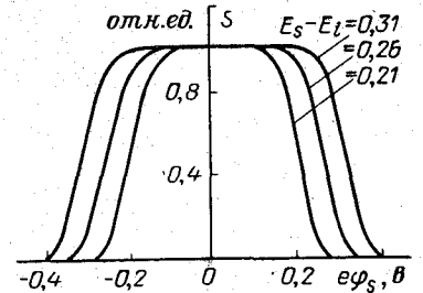
Рис. 9-9. Зависимость скорости поверхностной рекомбинации от поверхностного потенциала для различных значений E_s - E_i ( E_i — энергия, соответствующая середине запрещенной зоны).
