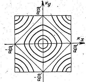
Рис. 2-10. Изоэнергетические поверхности для плоской квадратной решетки.
