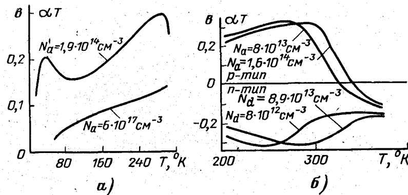
Рис. 5-5. Термо-э. д. с. германия при низких (а) и высоких (б) температурах.
