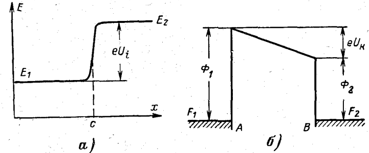
Рис. 8-6. Внутренняя (а) и внешняя (б) контактная разности потенциалов.
