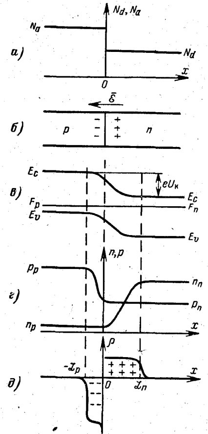
Рис. 8-12. Распределение примесей (а), разделение зарядов и возникновение электрического поля (б), зонная структура (в), распределение концентрации электронов и дырок (г) и распределение объемного заряда (д) в контакте электронного и дырочного полупроводников.
