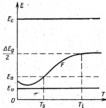
Рис. 3-13. Изменение положения уровня Ферми с температурой для акцепторного полупроводника.
