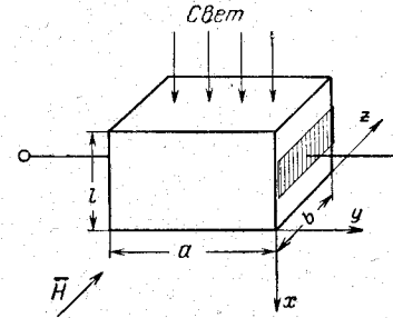
Рис. 11-12. Возникновение фотомагнитной э. д. с.
