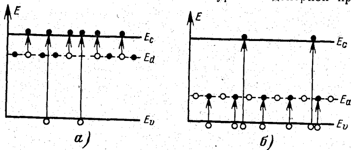
Рис. 1-10. Энергетическая диаграмма донорного (а) и акцепторного (б) полупроводников.
