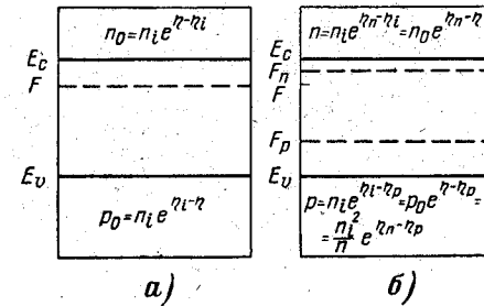
Рис. 6-2. Расщепление уровня Ферми на два квазиуровня — для электронов F_n и дырок F_p . а — равновесное состояние; б — неравновесное состояние.
