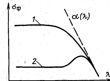
Рис. 11-8. Спектральная зависимость фотопроводимости (2) вблизи края фундаментального поглощения (1).
