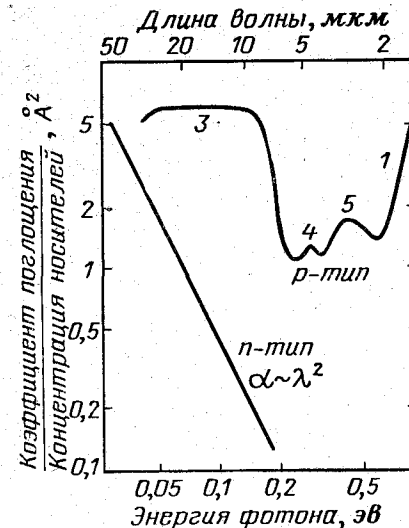
Рис. 10-14. Поглощение свободными носителями заряда в германии n - и p -типа.
