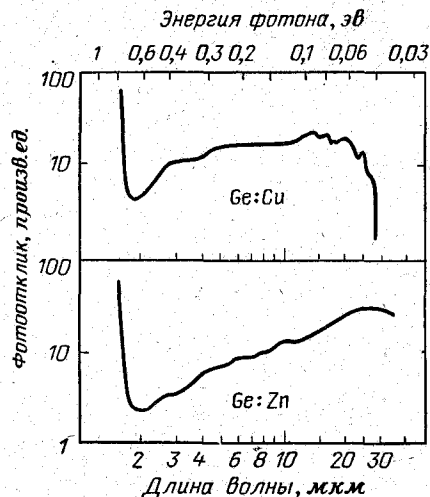
Рис. 11-10. Спектральные кривые фотопроводимости для кристаллов германия, легированных медью и цинком.
