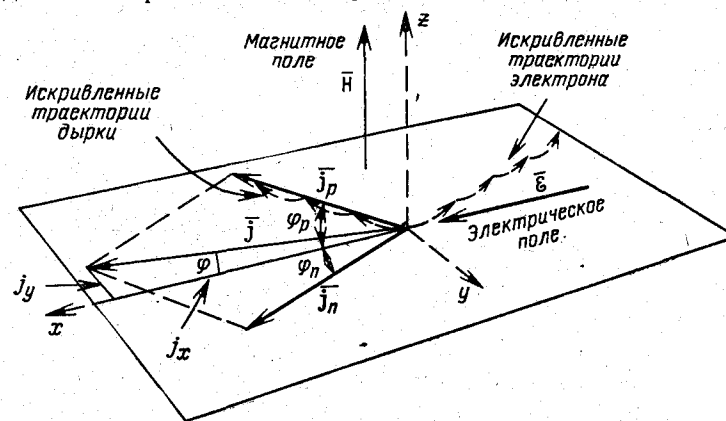
Рис. 1-14. Эффект Холла при наличии двух типов носителей заряда.
