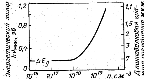
Рис. 10-6. Зависимости оптического энергетического зазора h\nu_{\text{мин}} от концентрации электронов в \text{InSb } n -типа.
