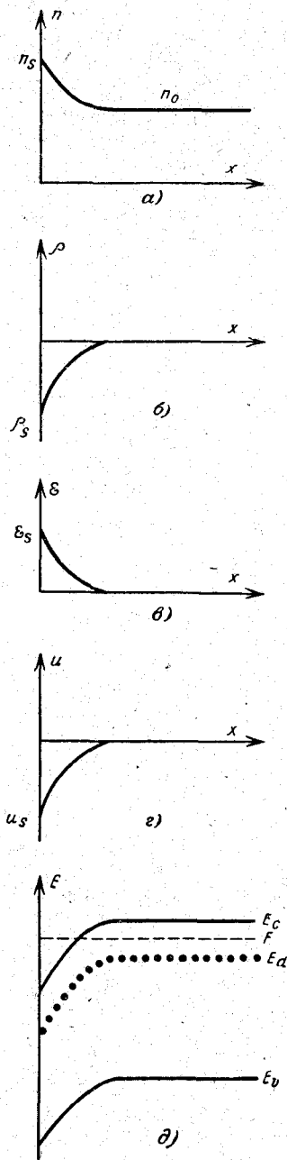
Рис. 8-2. Изменение концентрации свободных электронов (а), объемного заряда (б), поля (в), потенциальной энергии электронов (г) и искривление зон донорного полупроводника (д) во внешнем электрическом поле.
