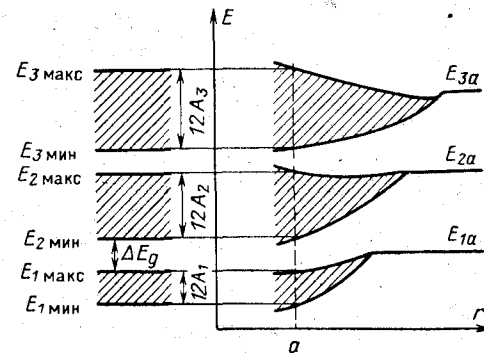
Рис. 2-3. Образование зон энергии из энергетических уровней при сближении атомов. a — постоянная решетки кристалла.
