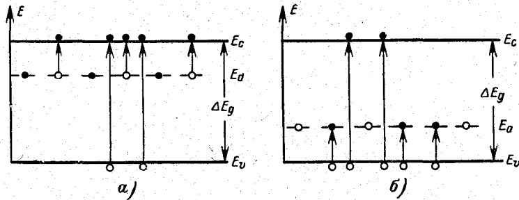
Рис. 3-2. Электронный (а) и акцепторный (б) полупроводники.
