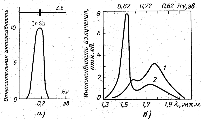
Рис. 10-20. Спектры рекомбинационного излучения антимида индия (а) и германия (б) при комнатной температуре. У германия экспериментальная кривая (2) дана с поправкой на самопоглощение.
