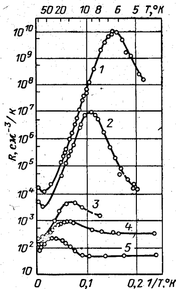
Рис. 3-16. Коэффициент Холла дырочных образцов германия как функция температуры при низких ее значениях.
