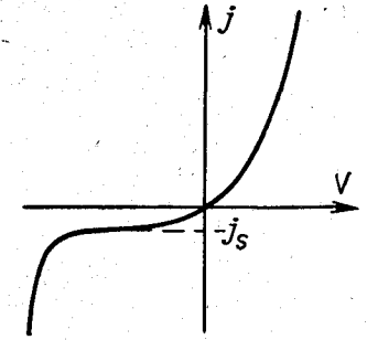
Рис. 8-14. Вольт-амперная характеристика p - n перехода.
