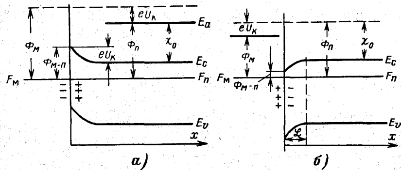
Рис. 8-7. Контакт металл — электронный полупроводник в случае (а) \Phi_m > \Phi_n и (б) \Phi_m < \Phi_n .
