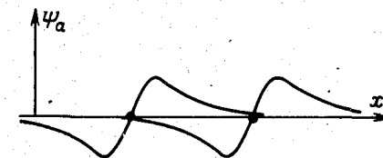
Рис. 2-7. Атомные функции p -состояния, описываемые уравнением (2-62).
