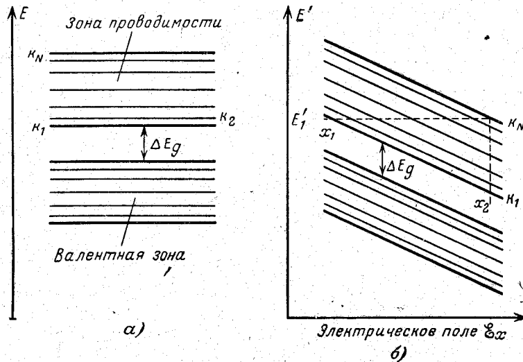
Рис. 2-11. Наклон энергетических зон во внешнем электрическом поле.
