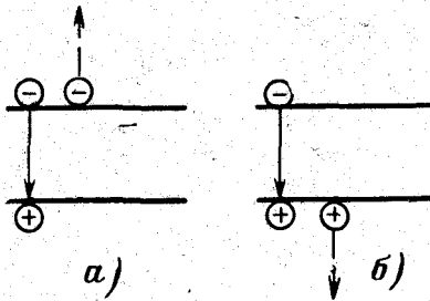
Рис. 6-4. Схема процессов ударной рекомбинации.
