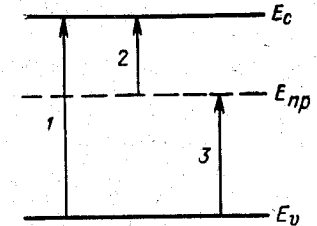
Рис. 11-1. Схема возможных оптических переходов электрона.
