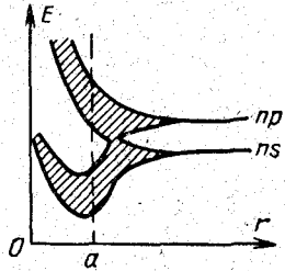
Рис. 4-14. Энергетическая схема атомного полупроводника.
