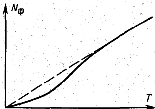
Рис. 4.13. Зависимость концентрации фононов от температуры.
