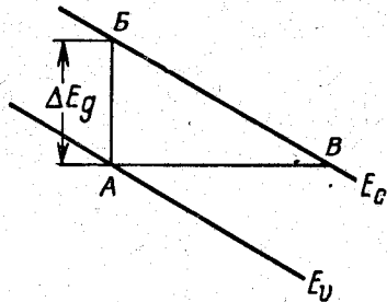
Рис. 5-15. Зонная структура беспримесного полупроводника при наличии сильного электрического поля.
