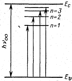
Рис. 10-11. Уровни энергии экситона.
