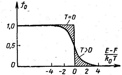
Рис. 3-1. Вид функции распределения Ферми — Дирака при T = 0 и T > 0 .
