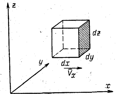
Рис. 4-1. Элементарный объем в геометрическом пространстве.
