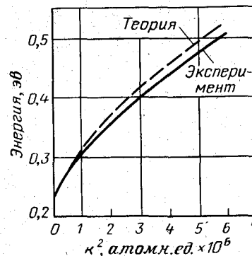
Рис. 2-19. Отклонение формы зоны проводимости в антиминоиде индия от параболической.
