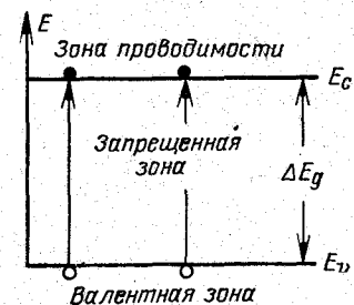
Рис. 1-8. Схематическое изображение энергетических зон собственного полупроводника.
