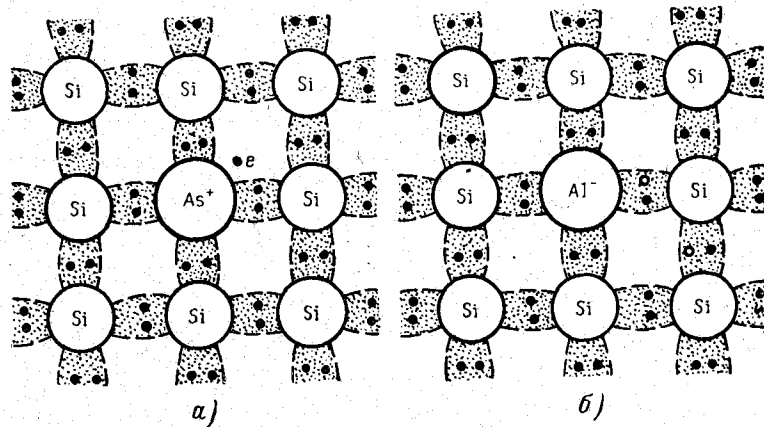
Рис. 1-9. Схематическое изображение кристаллической решетки донорного (а) и акцепторного (б) полупроводников.
