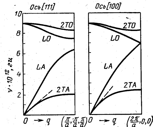
Рис. 4-12. Колебательный спектр решетки германия. TA и LA — поперечные и продольные акустические колебания, TO и LO — соответствующие оптические колебания.
