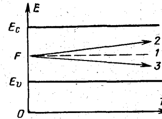
Рис. 3-6. Изменение уровня Ферми с температурой в собственном полупроводнике.
