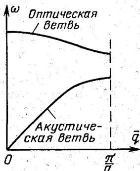
Рис. 4-11. Оптические и акустические ветви колебаний одномерной цепочки, в элементарной ячейке которой находятся два атома.
