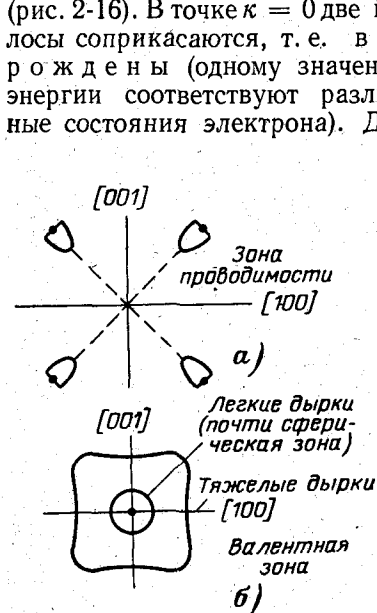
Рис. 2-17. Изоэнергетические поверхности в германии.
