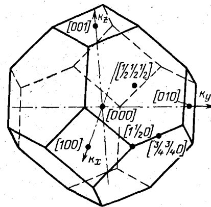
Рис. 2-15. Первая зона Бриллюэна полупроводника типа алмаза.
