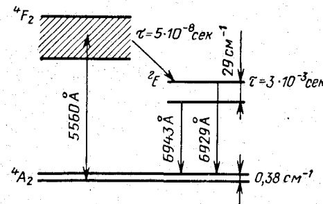
Рис. 10-22. Схема уровней в кристалле рубина.
