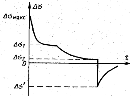
Рис. 9-6. Кривая релаксации поверхностной проводимости.
