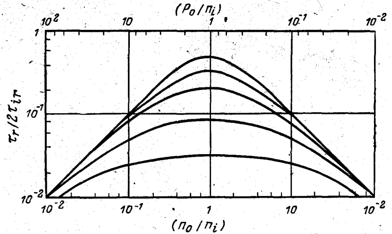
Рис. 6-3. Зависимость времени жизни для межзонной излучательной рекомбинации от концентрации носителей заряда при заданной температуре в случае низкого уровня возбуждения. В максимумах отношение \Delta n/n_i = 0 для верхней кривой, и соответственно равно 1, 3, 10, 30 для последующих кривых.
