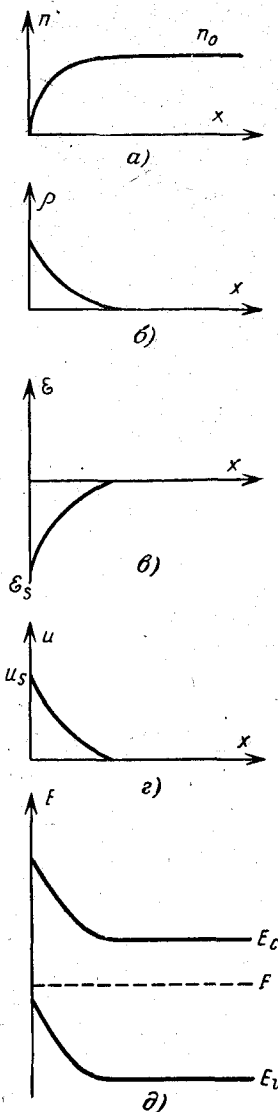
Рис. 8-3. Концентрация свободных электронов (а), объемный заряд (б), поле (в), потенциальная энергия электронов (г) и положение зон донорного полупроводника (д) при изменении направления внешнего электрического поля.
