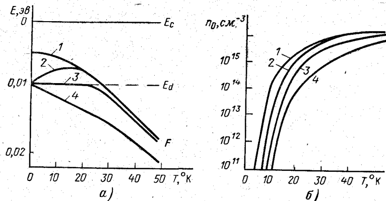
Рис. 3-14. Зависимость положения уровня Ферми (а) и концентрации электронов (б) от температуры при различной степени компенсации.
