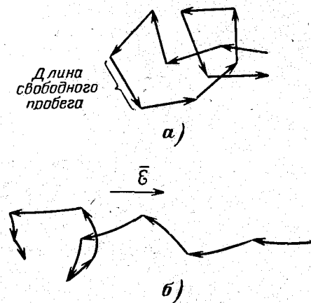
Рис. 1-6. Схема движения свободного электрона за счет тепловой энергии (а) и во внешнем электрическом поле (б).
