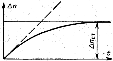
Рис. 11-3. Изменение во времени концентрации носителей заряда при освещении.
