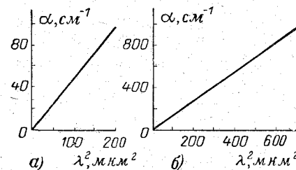
Рис. 10-13. Зависимость поглощения электронами проводимости в сурьмянистом индии n -типа от \lambda^2 для концентрации электронов 3,5 \cdot 10^{17} \text{ см}^{-3} (а) и 6,2 \cdot 10^{17} \text{ см}^{-3} (б).
