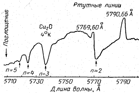
Рис. 10-12. Спектр экситонного поглощения в закиси меди.
