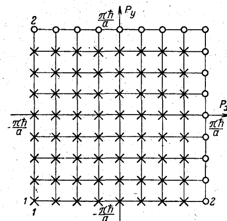
Рис. 2-5. Сечение первой зоны Бриллюэна для простой кубической решетки плоскостью P_z = 0 .
