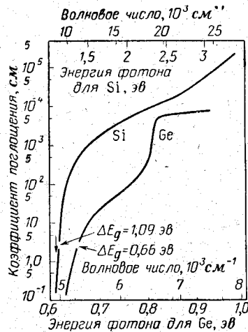
Рис. 10-8. Спектр поглощения германия и кремния.
