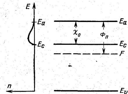
Рис. 8-4. Работа выхода электронов из полупроводника.
