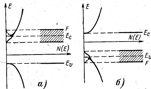
Рис. 3-19. Плотность состояний и положение уровня Ферми в вырожденном электронном (а) и дырочном (б) полупроводниках.
