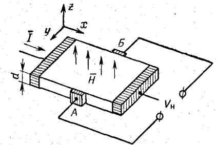
Рис. 1-11. Образец для измерения эффекта Холла.
