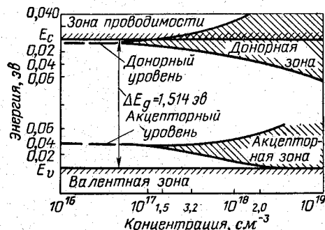
Рис. 3-18. Появление донорной и акцепторной зон в арсениде галлия и их слияние с зоной проводимости и валентной при увеличении концентрации примеси.
