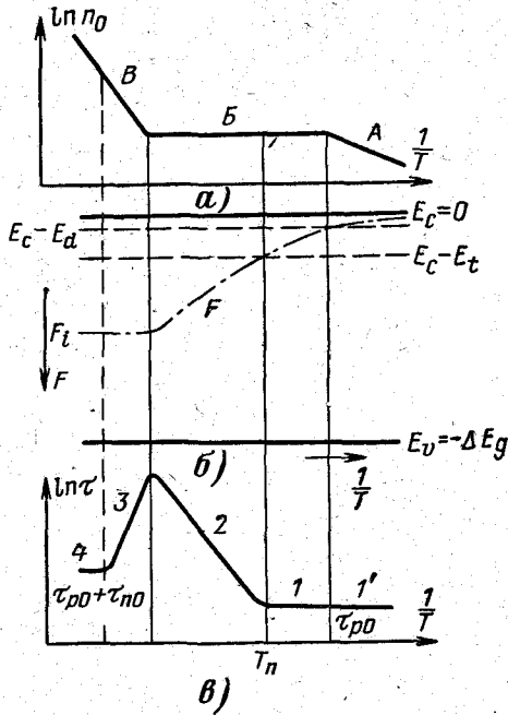
Рис. 6-8. Зависимость равновесной концентрации (а), уровня Ферми (б) и времени жизни (в) от температуры для донорного полупроводника.
