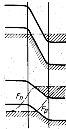
Рис. 10-23. Вырожденный p - n переход в равновесном состоянии и при приложении напряжения в пропускном направлении.
