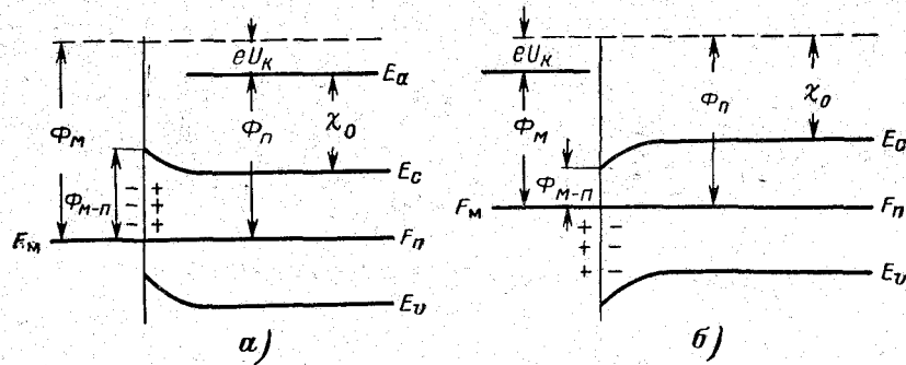
Рис. 8-9. Контакт металл — собственный полупроводник в случае (а) \Phi_m > \Phi_n и (б) \Phi_m < \Phi_n .
