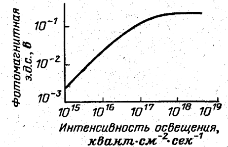
Рис. 11-14. Зависимость фотомангнитной э. д. с. от интенсивности освещения для германия.
