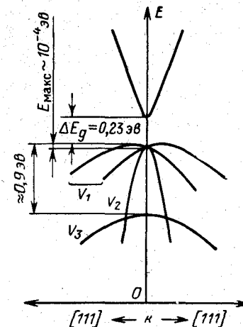
Рис. 2-20. Энергетическая структура антиминоида индия.
