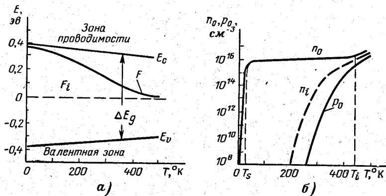
Рис. 3-12. Температурная зависимость уровня Ферми (а) и концентрации (б) носителей заряда для германия, легированного сурьмой.
