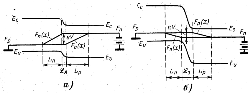
Рис. 8-16. Квазиуровень Ферми в p - n переходе при прямом (а) и обратном (б) смещении.
