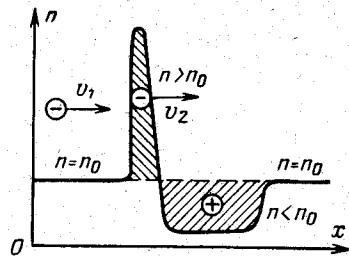
Рис. 5-11. Структура электрического домена.
