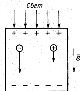
Рис. 11-11. Возникновение э. д. с. Дембера.
