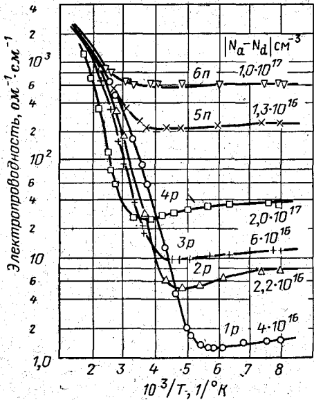
Рис. 5-3. Зависимость электропроводности от обратной температуры для двух n-типа и четырех p-типа образцов InSb.
