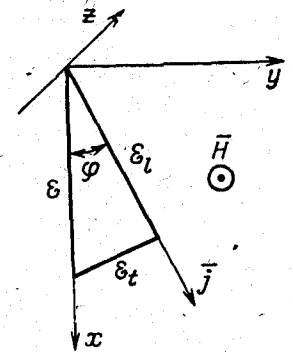
Рис. 1-13. К выводу выражения для коэффициента Холла.
