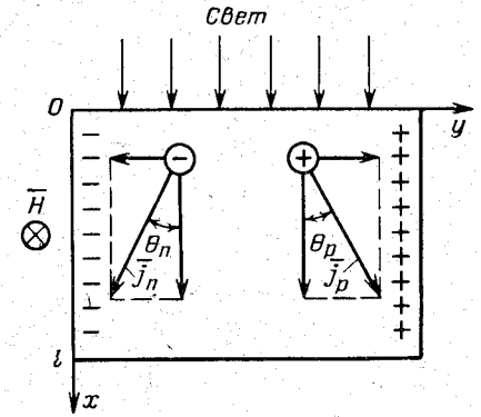
Рис. 11-13. Действие магнитного поля на диффузионные токи электронов и дырок.
