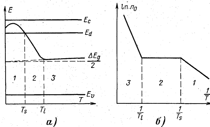
Рис. 3-11. Изменение положения уровня Ферми (а) и концентрации электронов (б) с температурой для донорного полупроводника.
