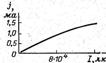
Рис. 11-17. Люкс-амперная характеристика германиевого фотодиода.
