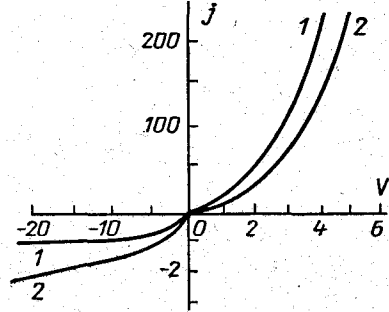
Рис. 8-11. Вольт-амперные характеристики контакта металл — полупроводник.
