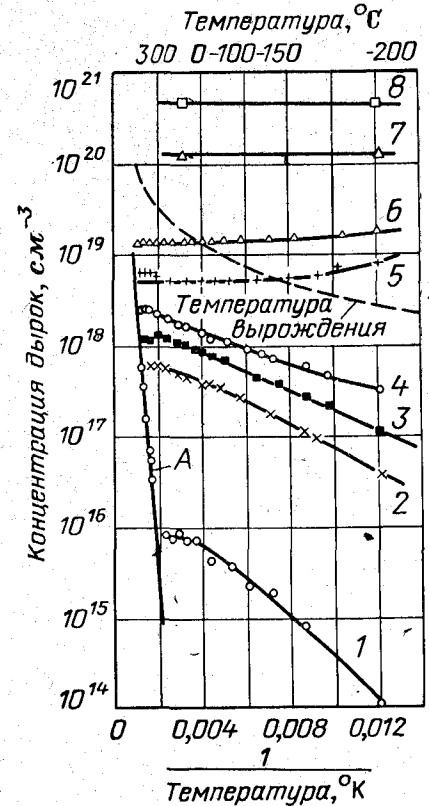
Рис. 3-4. Температурная зависимость концентрации дырок в кремнии, легированном бором. А — собственная концентрация. Концентрация атомов бора для различных кривых равна ( \text{см}^{-3} ): 1 — нелегированный; 2 — 6,7 \cdot 10^{17} ; 3 — 1,3 \cdot 10^{18} ; 4 — 2,7 \cdot 10^{18} ; 5 — 6,7 \cdot 10^{18} ; 6 — 1,3 \cdot 10^{19} ; 7 — 1,3 \cdot 10^{20} ; 8 — 1,3 \cdot 10^{21} . Пунктирная кривая показывает связь концентрации дырок с температурой, при которой наступает вырождение.
