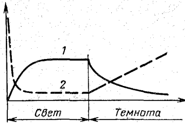
Рис. 11-5. Релаксация неравновесной концентрации электронов (1) и их мгновенное время жизни (2) для случая квадратичной рекомбинации.
