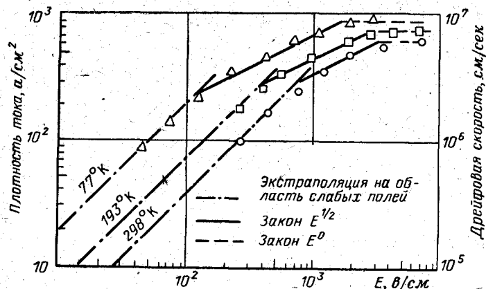
Рис. 5-7. Зависимость плотности тока от напряженности электрического поля в электронном германии.
