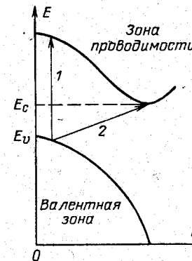
Рис. 11-2. Прямые (1) и непрямые (2) оптические межзонные переходы.
