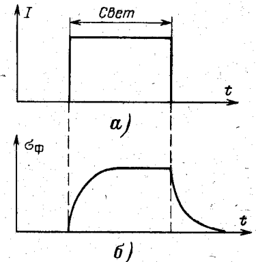
Рис. 11-4. Релаксация неравновесной проводимости (б) при возбуждении прямоугольным импульсом света (а).
