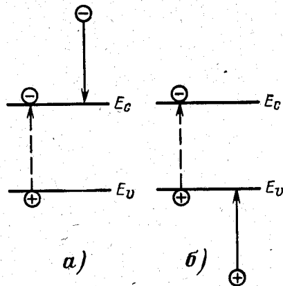
Рис. 5-13. Два возможных варианта ударной ионизации.
