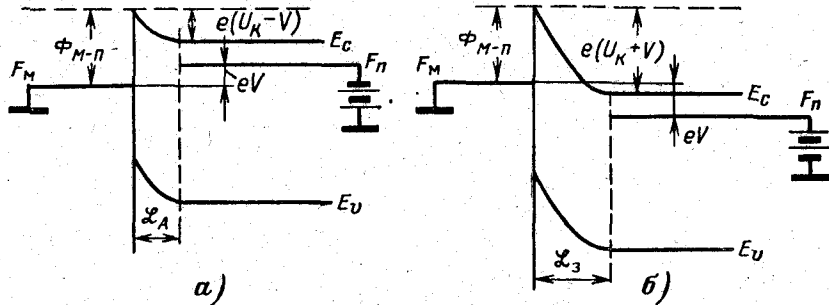
Рис. 8-10. Прямое (а) и обратное (б) подключение батареи к контакту металл — полупроводник.
