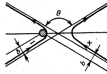
Рис. 4-3. Искривление траектории движения электрона в поле положительного иона примеси.
