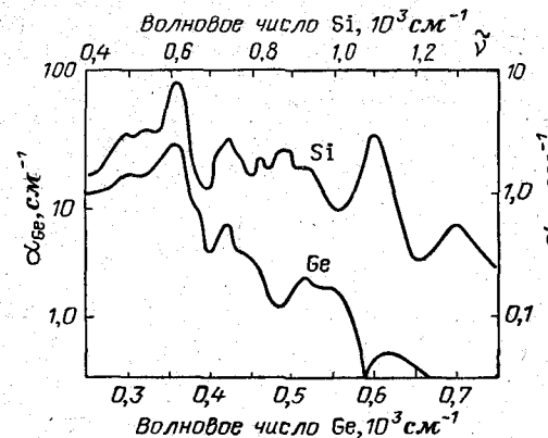
Рис. 10-16. Поглощение решеткой германия и кремния.
