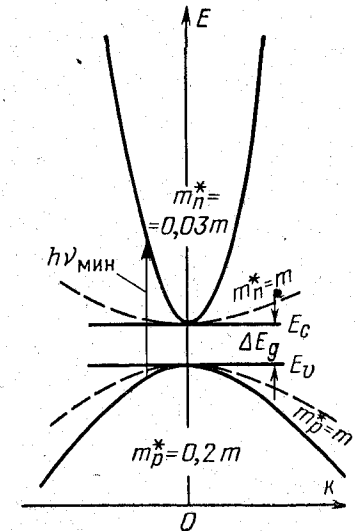
Рис. 10-7. Зависимость энергии от квазиимпульса в антимониде индия.
