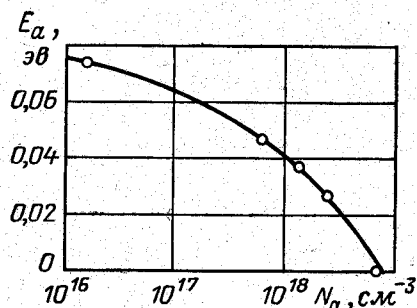
Рис. 3-17. Зависимость энергии ионизации атомов бора от его концентрации в кремнии.
