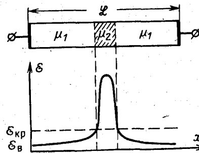
Рис. 5-10. Распределение электрического поля вдоль образца.
