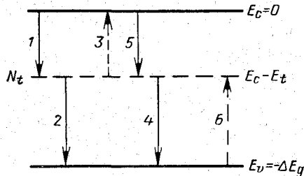
Рис. 6-6. Переходы электронов, связанные с рекомбинацией через локальные центры.
