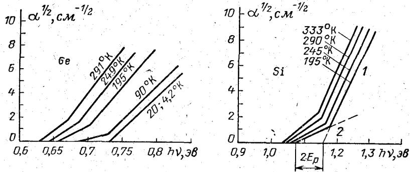
Рис. 10-10. Зависимость \alpha^{1/2} от температуры для германия и кремния.
