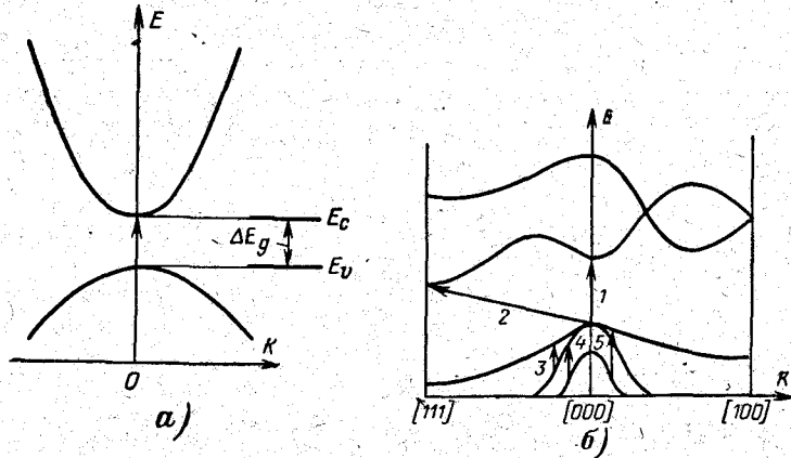
Рис. 10-2. Собственное поглощение при прямых межзонных переходах (а) и оптические переходы в полупроводнике со сложными энергетическими зонами (б).
