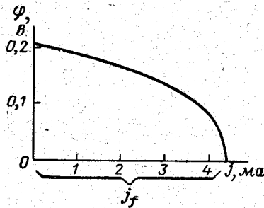
Рис. 11-16. Вольт-амперная характеристика германиевого фотодиода в вентильном режиме.
