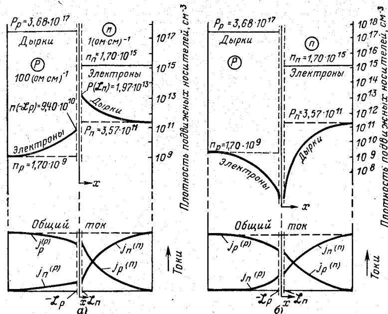
Рис. 8-15. Концентрации носителей заряда и токов в p - n переходе при прямом (а) и обратном (б) смещении.
