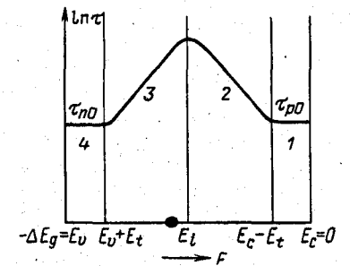
Рис. 6-7. Изменение времени жизни в зависимости от положения уровня Ферми.
