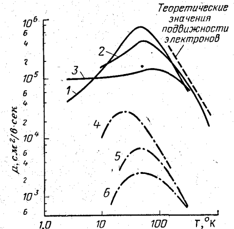
Рис. 5-2. Температурные зависимости подвижности электронов и дырок в InSb. 1 — n = 2 \cdot 10^{14} ; 2 — n = 10^{15} ; 3 — n = 10^{16} ; 4 — p = 3 \cdot 10^{14} ; 5 — p = 4 \cdot 10^{15} и 6 — p = 3 \cdot 10^{16} \text{ см}^{-3} .
