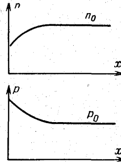
Рис. 9-3. Распределение концентрации электронов и дырок в глубине и в приповерхностном слое полупроводника n -типа.
