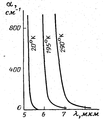
Рис. 10-5. Спектр поглощения антимонида индия при разных температурах.
