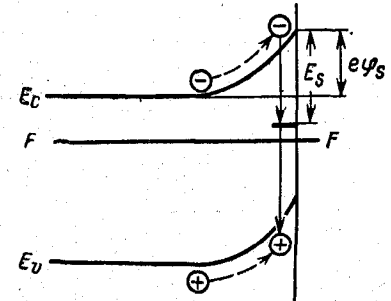
Рис. 9-8. Рекомбинация через поверхностные уровни.
