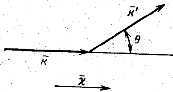
Рис. 4-2. Изменение волнового вектора электрона при рассеянии.
