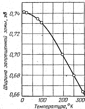
Рис. 3-8. Температурная зависимость ширины запрещенной зоны германия.
