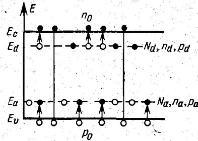
Рис. 3-10. Полупроводник, имеющий примеси донорного и акцепторного типа.
