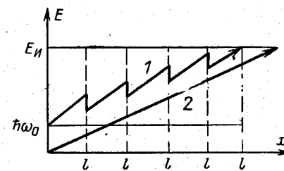
Рис. 5-14. Условная диаграмма ударной ионизации.
