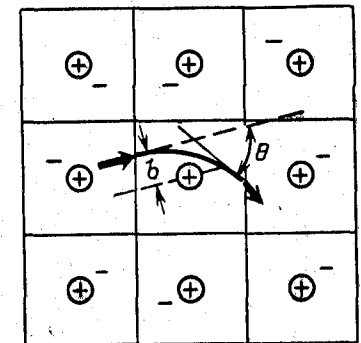
Рис. 4-4. Рассеяние электрона и дырки на положительном ионе примеси.
