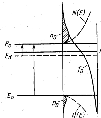
Рис. 6-1. Тепловая генерация свободных носителей и их концентрация в состоянии термодинамического равновесия.
