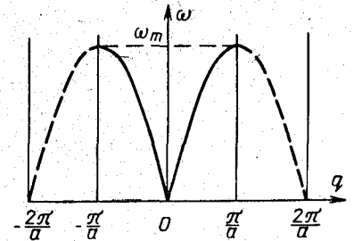
Рис. 4-7. Зависимость частоты колебаний от волнового числа для линейной решетки, состоящей из одинаковых атомов.
