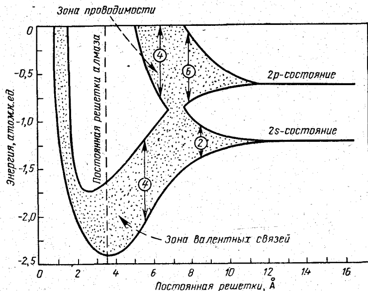
Рис. 2-4. Образование энергетических зон из атомных уровней в алмазе.
