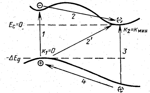
Рис. 10-9. Непрямые оптические переходы электрона из валентной зоны в зону проводимости.
