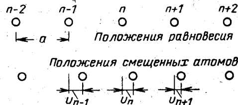
Рис. 4-6. Схематическое изображение линейной решетки одинаковых атомов.
