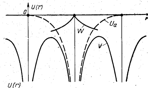
Рис. 2-1. Схематическое изображение периодического потенциала одномерной решетки.
