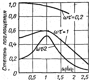
Рис. 2-13. Степень поглощения при циклотронном резонансе в зависимости от напряженности постоянного магнитного поля (в единицах \omega/\omega_c ).
