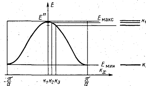
Рис. 2-8. Зависимость E(k_x) для p -состояния.
