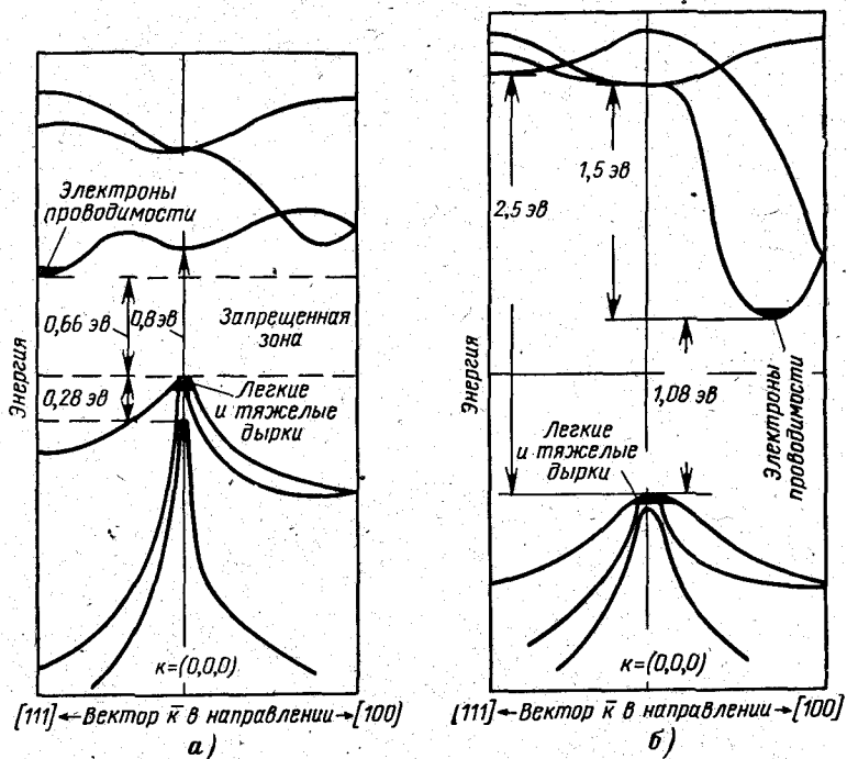
Рис. 2-16. Энергетическая структура германия (а) и кремния (б).
