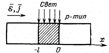
Рис. 7-4. Одномерная модель полупроводникового образца.
