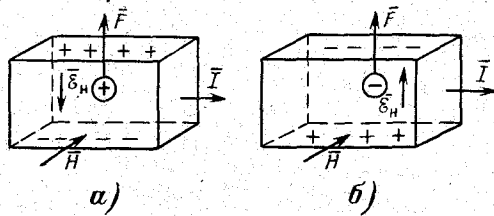
Рис. 1-12. Отклонение носителей заряда под воздействием магнитного поля в образцах с дырочной (а) и электронной (б) проводимостью.
