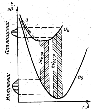
Рис. 10-18. Схема энергетических уровней примесного центра в твердом теле.
