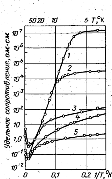
Рис. 3-15. Удельное сопротивление дырочных образцов германия как функция температуры при низких ее значениях.
