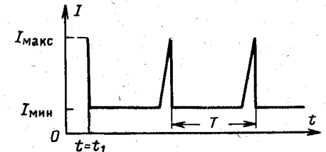
Рис. 5-12. Эпюра тока через образец арсенида галлия.
