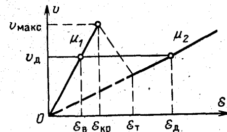
Рис. 5-9. Зависимость скорости движения носителей заряда в арсениде галлия от напряженности поля в образце.
