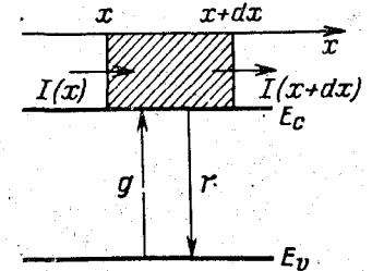
Рис. 7-1. К выводу уравнения непрерывности.
