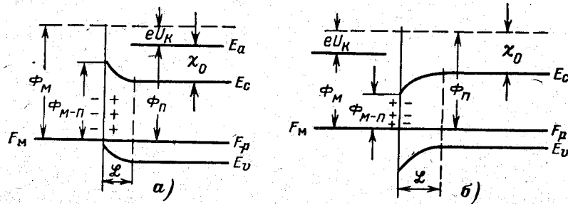
Рис. 8-8. Контакт металл — дырочный полупроводник в случае (а) \Phi_M > \Phi_n и (б) \Phi_M < \Phi_n .
