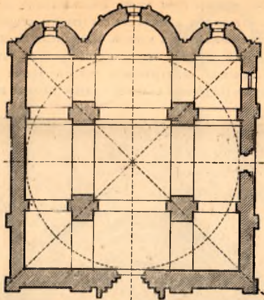
6. Церковь Пантелеймона в Галиче. План
