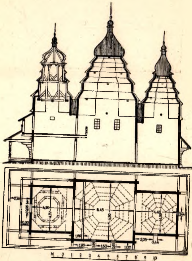
44. Храм в с. Кривках. План и разрез
