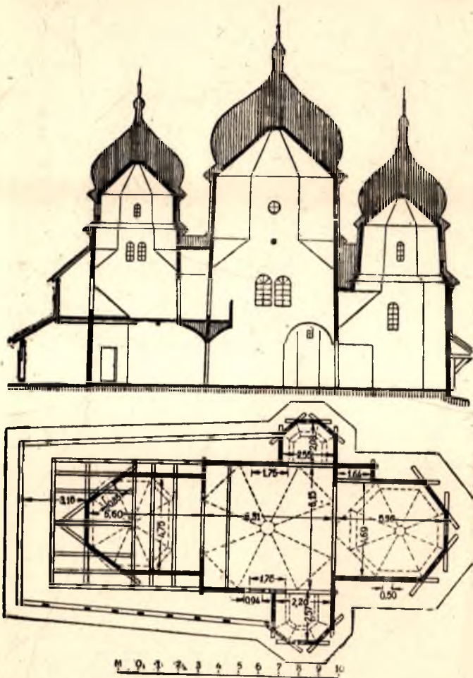
46. Храм в Дрогобыче. План и разрез
