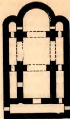
9. Церковь Богородицы в Галиче. План абсиды
