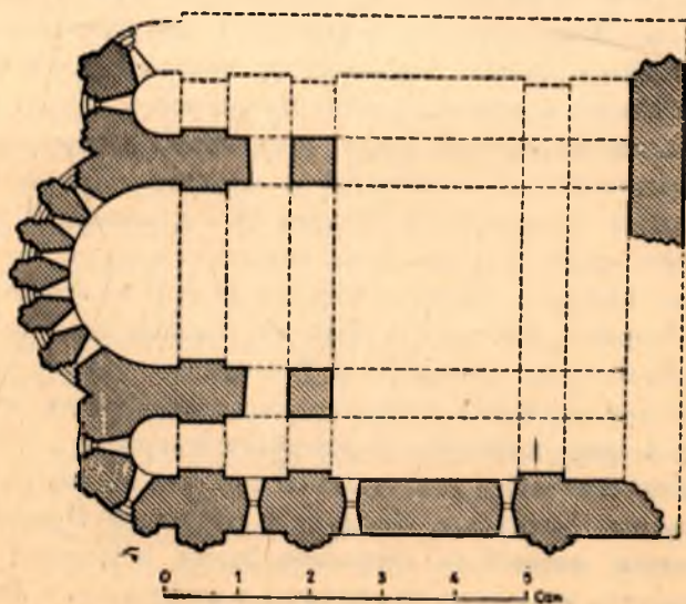
3. Храм Василия в Овруче. План
