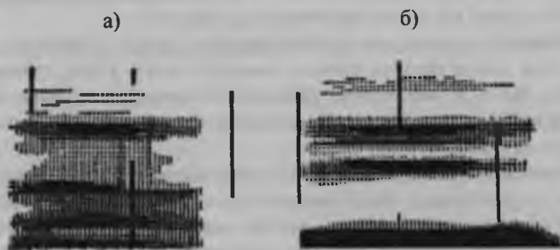
Мал. 7. Спектрограми.
