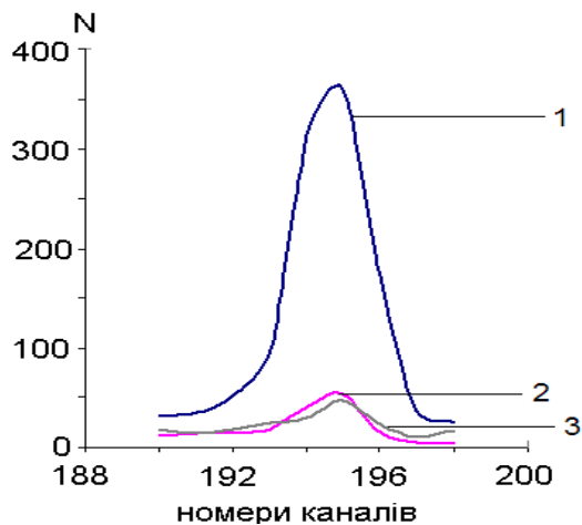
Рис. 5. Максимуми у межах 192 - 198 каналів, що зумовлені випромінюванням ^{137m}\text{Ba} , сорбованого ФТ: 1–пік ^{137m}\text{Ba} на поверхні фосфату титану, через 4,1 хв після завершення опромінювання; 2–пік ^{137m}\text{Ba} на поверхні фосфату титану, через 13хв після завершення опромінювання; 3–ділянка гамма-спектру опроміненого фосфату титану без сорбованого барію.
