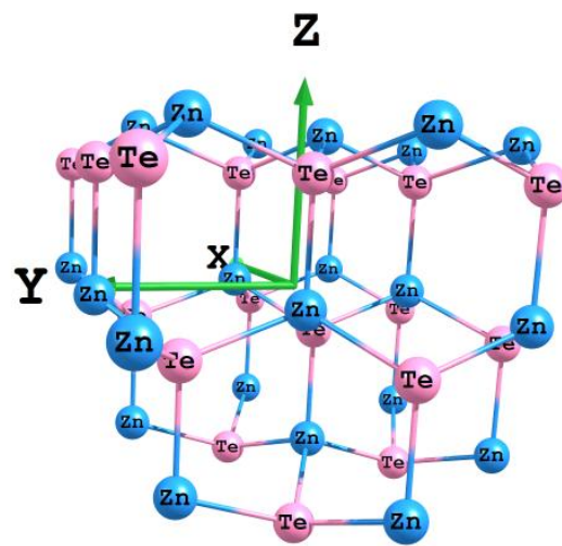
Рис. 2. Структура вюрцитної модифікації α-ZnTe Ошибка! Источник ссылки не найден.
