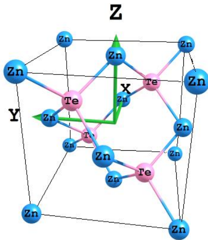
Рис. 1. Структура сфалеритної модифікації кристалів β-ZnTe Ошибка! Источник ссылки не найден.
