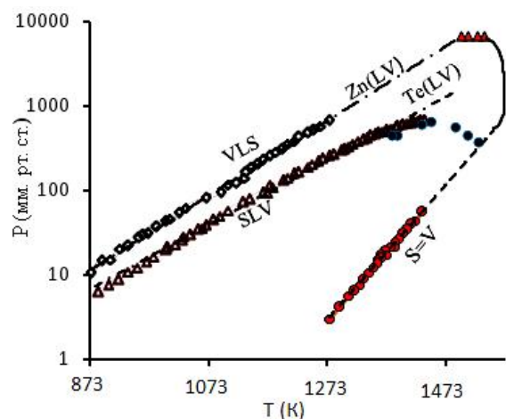
Рис. 5. P-T проекція фазової діаграми системи Zn-Te. Незаповнені символи (VLS, SLV, і S=V ) – експериментальні результати Ошибка! Источник ссылки не найден. ; заповнені символи (VLS, SLV, і S=V ) – експериментальні результати Ошибка! Источник ссылки не найден.
