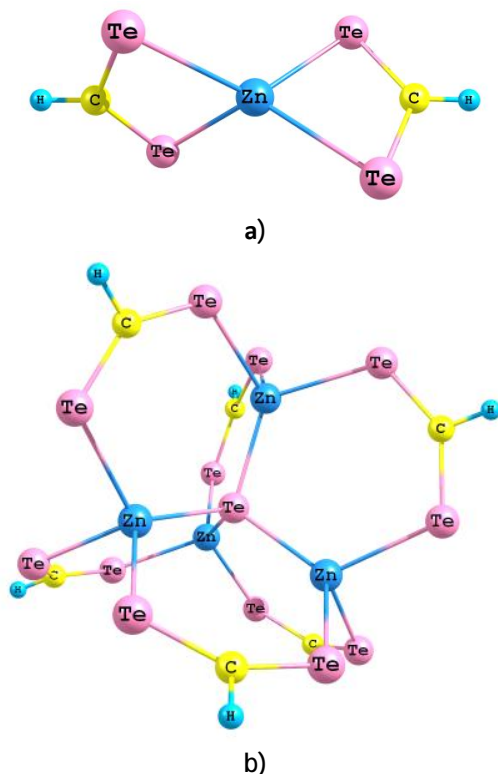
Рис. 6. Модель кластерів А ( \text{ZnC}_2\text{H}_2\text{S}_4 ) (а) і В ( \text{Zn}_4\text{C}_6\text{H}_6\text{S}_{13} ) (b) відповідно для кубічної фази \beta -ZnTe.
