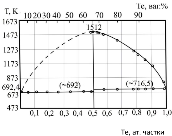
Рис. 3. T-x-діаграма рівноваги системи Zn-Te Ошибка! Источник ссылки не найден.
