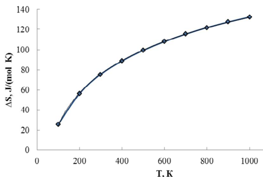
Рис. 10. Температурна залежність ентропії \Delta S для кристалів \text{ZnTe} : лінія – апроксимація аналітичною функцією (25), точки – квантово-хімічний
