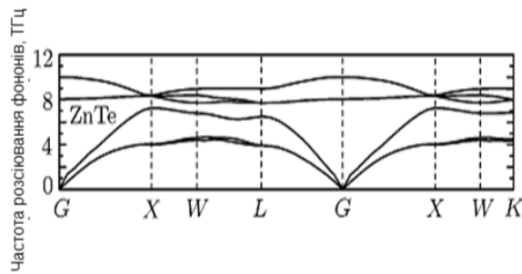
Рис. 7. Фононний спектр для характерних точок зони Бріллюена у кристалах ZnTe Ошибка!
