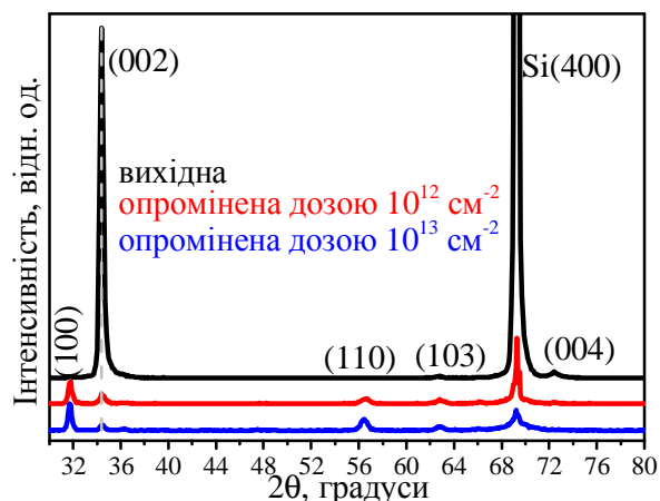
Рис. 1. Рентгенограма вихідних та опроміненних іонами He^{26+} плівок ZnO, осаджених на підкладки n-кремнію.
