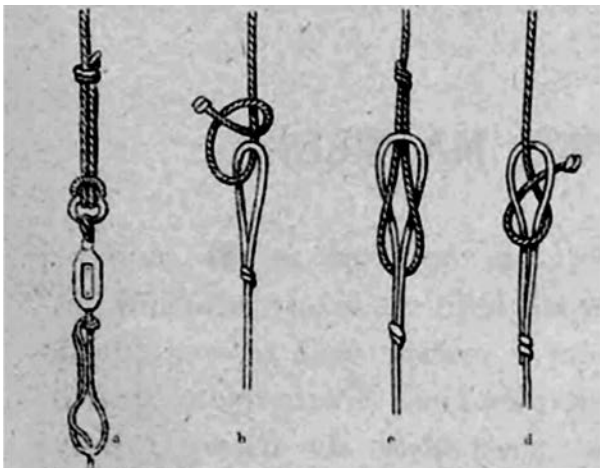
Fig. 84. Wiązanie sznurka wędki z przezroczystą częścią z haczykiem.
