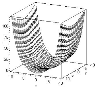
Рис. 10. Графік функції |\text{Chc } z|
