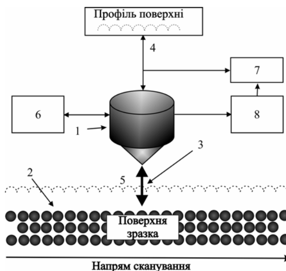
Рис.1. Принцип роботи скануючого зондового мікроскопа: 1-зонд; 2-окремий атом; 3-фізична характеристика (тунельний струм, міжатомні сили і т.п.); 4-вихідний сигнал; 5-траєкторія руху зонда; 6- коло керування процесом сканування; 7- коло зворотнього зв'язку; 8- коло детектування досліджуваної фізичної характеристики [1].
